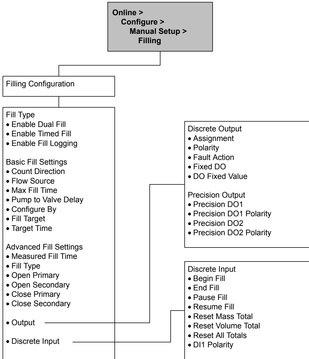
Abbildung C-7: Menü Abfüllung
