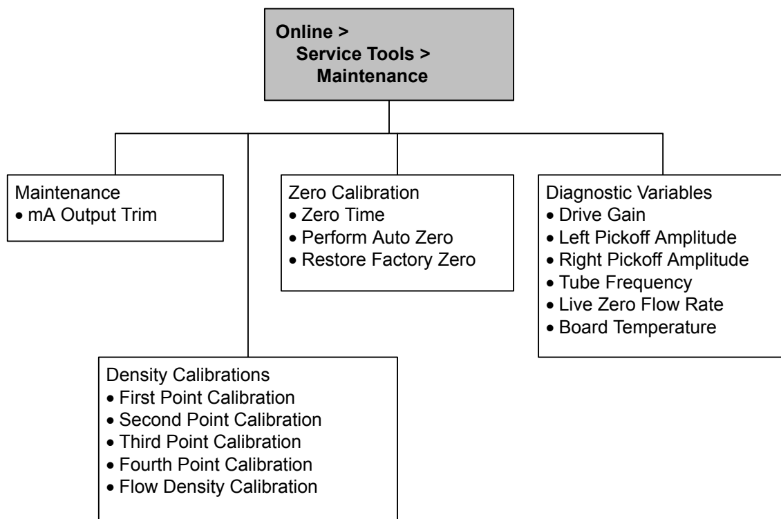
Abbildung C-10: Menü Wartung
