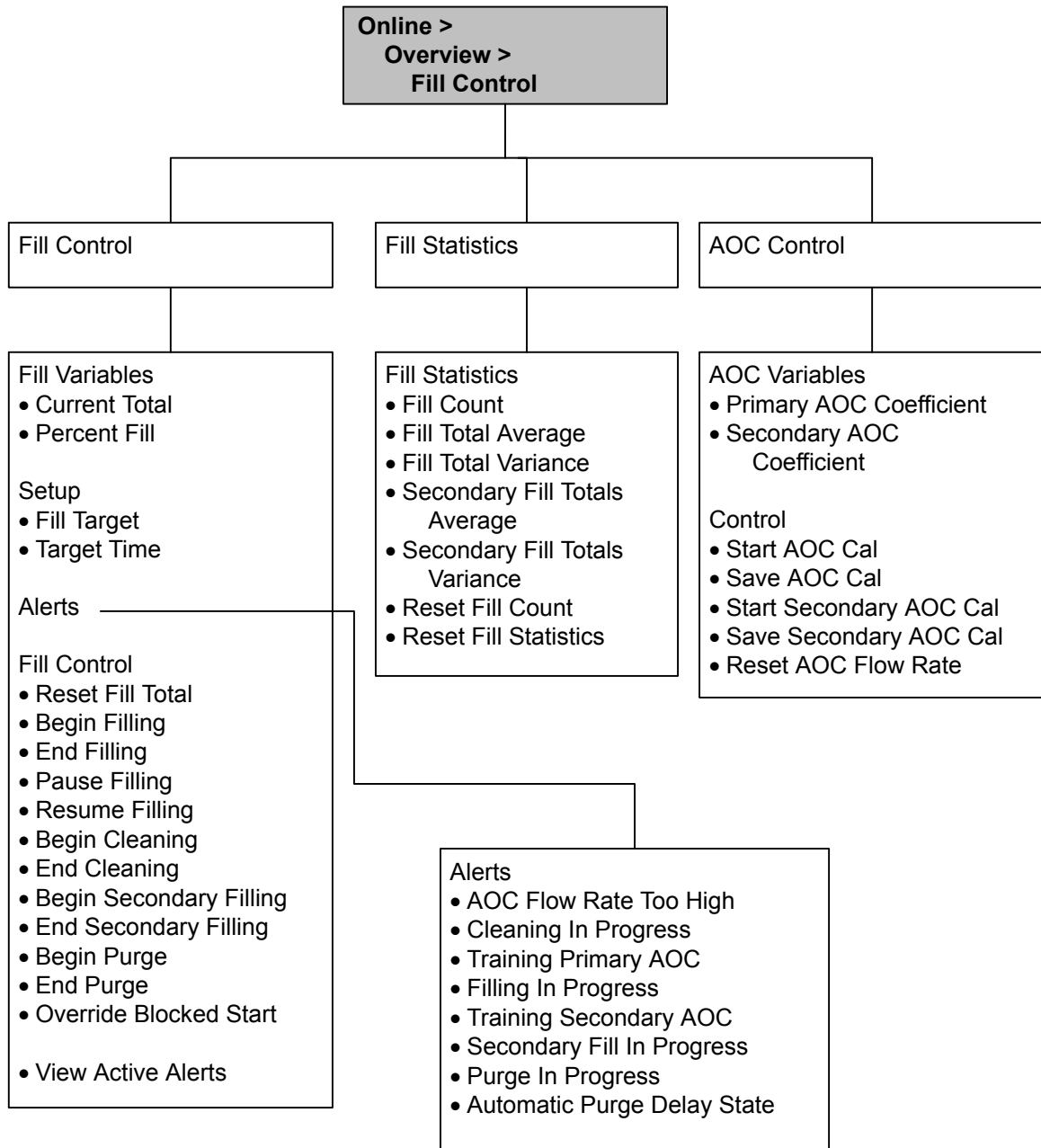
Abbildung C-3: Menü Abfüllsteuerung
