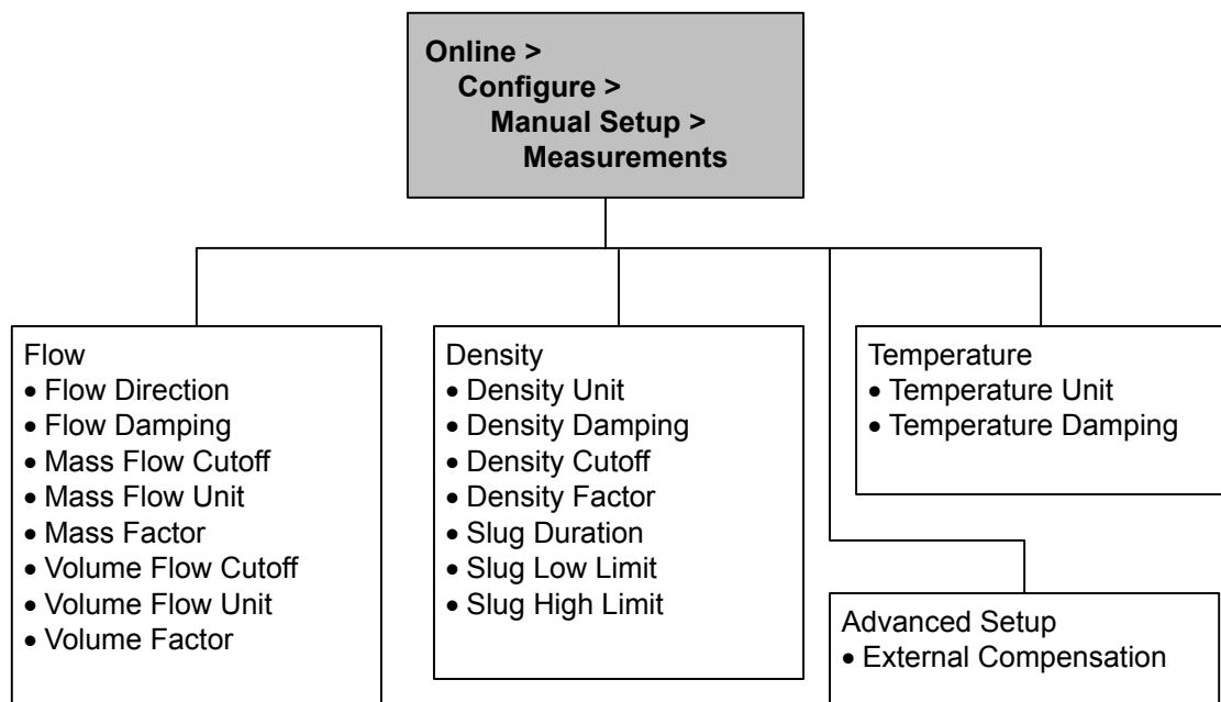
Abbildung C-6: Menü Messungen
