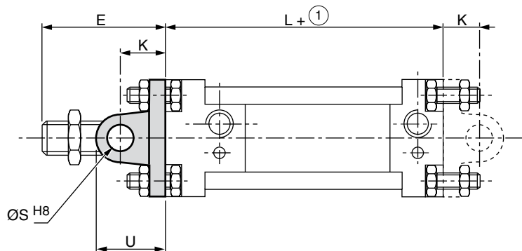
MONTAJE Horquilla hembra CNOMO 06-07-14
