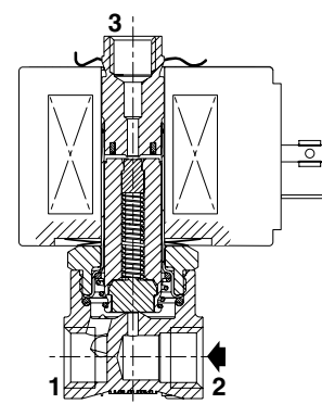
NC function (1/8)
