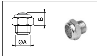
Protector de escape (acero inoxidable)
