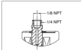
Escape superior del piloto baja potencia (Interfaz de solenoide ASCO)
