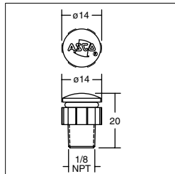
Protector de escape del piloto Número de pieza 276405-001
