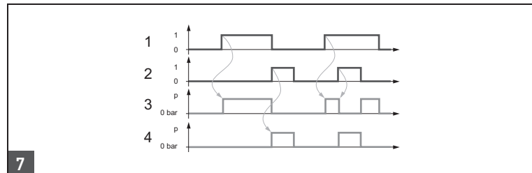
7 Comando varianti eiettori NC / Pilotaje variante de eyector NC / Styrning ejektorvariant NC 1 = "Aspirazione" [IN 1] / "Aspiración" [IN 1] / "Undertryck" [IN 1] 2 = "Scarico" [IN 2] / "Purga" [IN 2] / "Lossblås" [IN 2] 3 = Stato "Aspirazione" / Estado "Aspiración" / Status "Undertryck" 4 = Stato "Scarico" / Estado "Purga" / Status "Lossblås"
