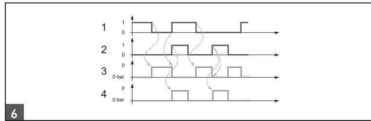
6 Comando varianti eiettori NO / Pilotaje variante de eyector NO / Styrning ejektorvariant NO 1 = "Aspirazione" [IN 1] / "Aspiración" [IN 1] / "Undertryck" [IN 1] 2 = "Scarico" [IN 2] / "Purga" [IN 2] / "Lossblås" [IN 2] 3 = Stato "Aspirazione" / Estado "Aspiración" / Status "Undertryck" 4 = Stato "Scarico" / Estado "Purga" / Status "Lossblås"
