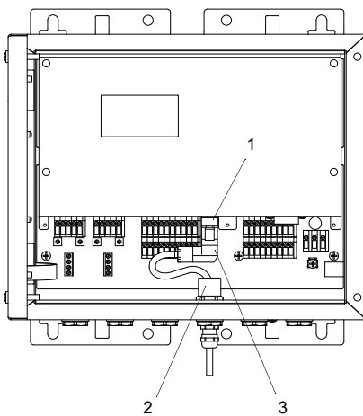
Abb. 8.24: Anschluss des LAN-Kabels
