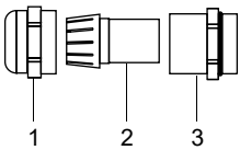
Abb. 8.15: Kabelverschraubung für Aluminiumgehäuse
