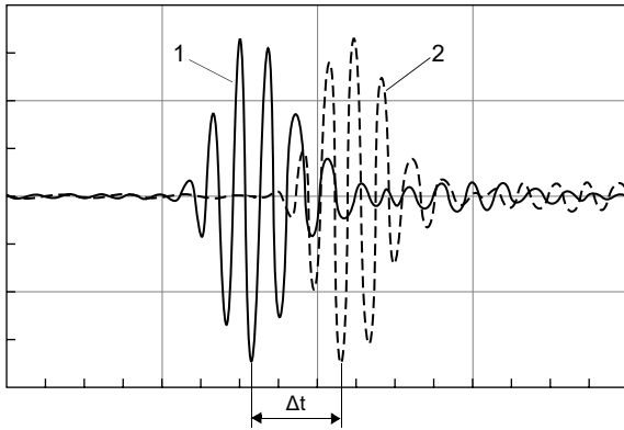
Abb. 4.3: Laufzeitdifferenz \Delta t
