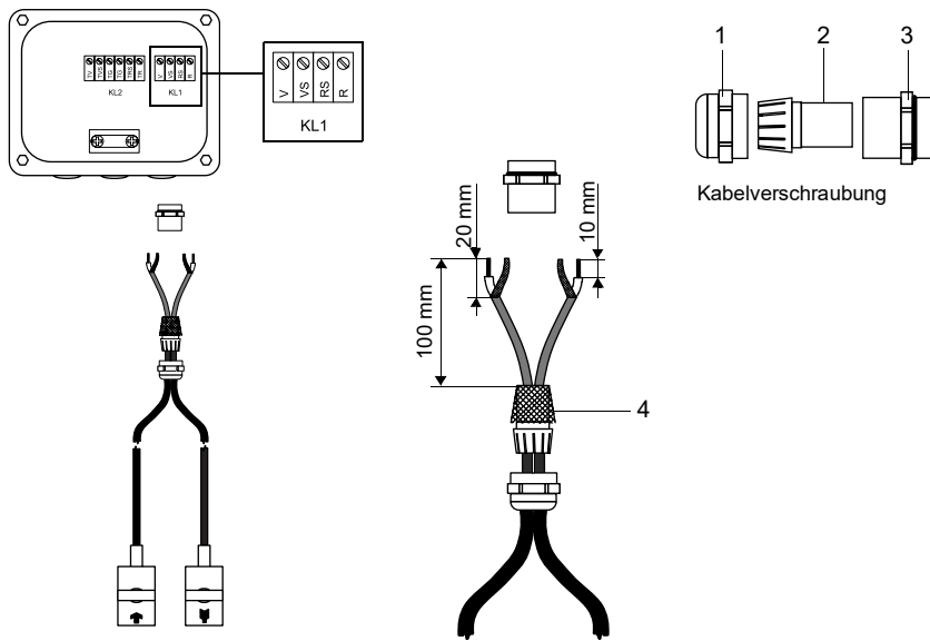
Abb. 8.7: Anschluss des Sensorkabels mit Kunststoffkabelmantel und abisolierten Kabelenden
