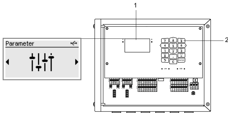
Abb. 5.2: Bedienungsfeld des Messumformers
