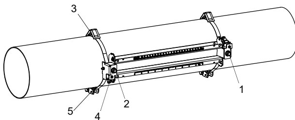
Abb. 7.50: Schiene am Rohr
