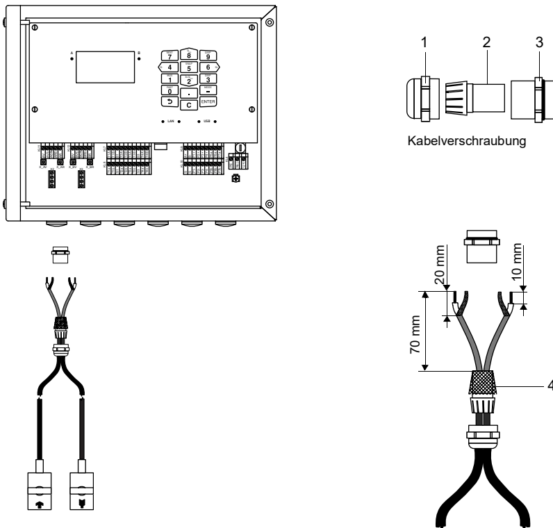
Abb. 8.3: Anschluss des Sensorkabels mit Kunststoffkabelmantel und abisolierten Kabelenden an den Messumformer
