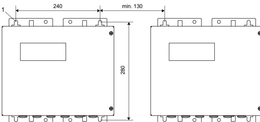
Abb. 7.3: Messumformer (Abmessungen in mm)
