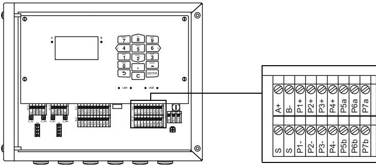
Abb. 8.16: Anschluss der Ausgänge am Messumformer
