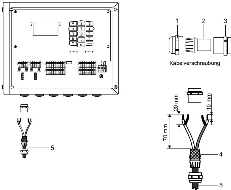
Abb. 8.5: Anschluss des Verlängerungskabels an den Messumformer
