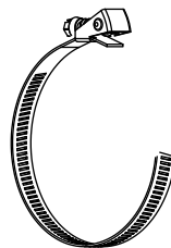
Abb. 7.40: Schnellspannschloss mit Spannband
