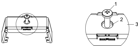
Abb. 7.56: Federbügel
