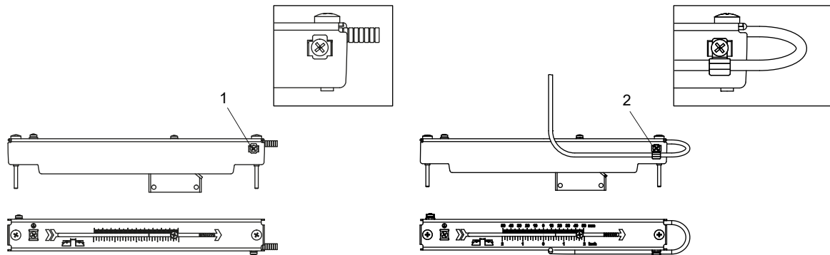
Abb. 7.33: Fixieren der Sensorkabel
