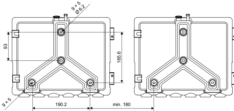
Abb. 7.4: Messumformer (Abmessungen in mm)
