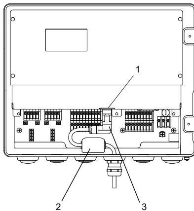
Abb. 8.26: Anschluss des LAN-Kabels
