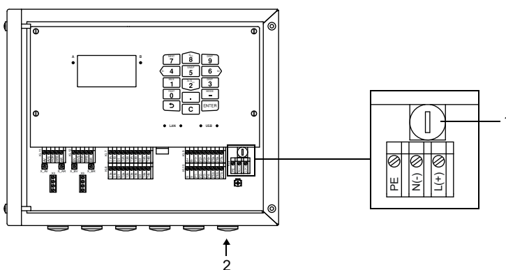
Abb. 8.13: Anschluss der Spannungsversorgung am Messumformer
