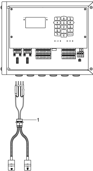
Abb. 8.4: Anschluss des Sensorkabels mit Edelstahlmantelung und abisolierten Kabelenden an den Messumformer
