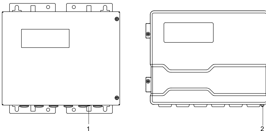
Abb. 8.12: Potentialausgleichsklemme am Messumformer
