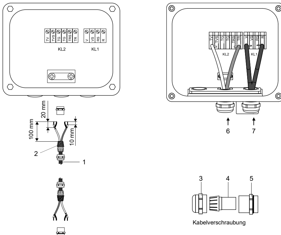
Abb. 8.9: Anschluss des Verlängerungskabels an das Klemmengehäuse (ohne Potentialtrennung)
