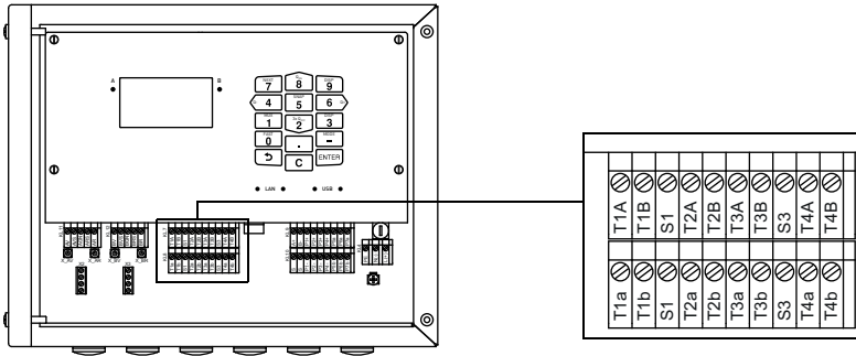
Abb. 8.17: Anschluss der Eingänge am Messumformer
