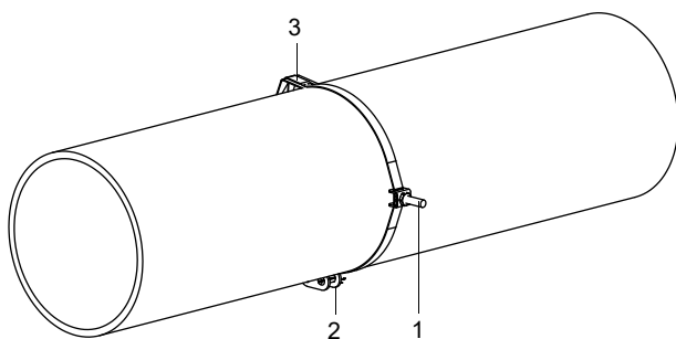
Abb. 7.17: Spannband mit Spannbandklammer und Metallfeder am Rohr
