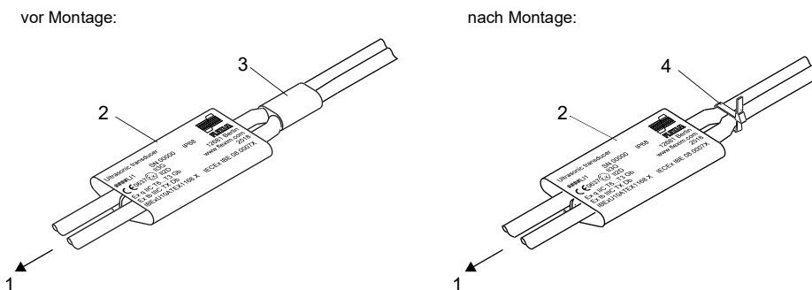
Abb. 7.10: Typenschild am Sensorkabel
