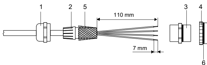
Abb. 8.19: Konfektionierung des Temperaturfühlers
