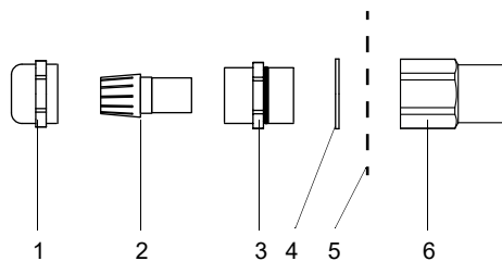
Abb. 8.14: Kabelverschraubung für Edelstahlgehäuse
