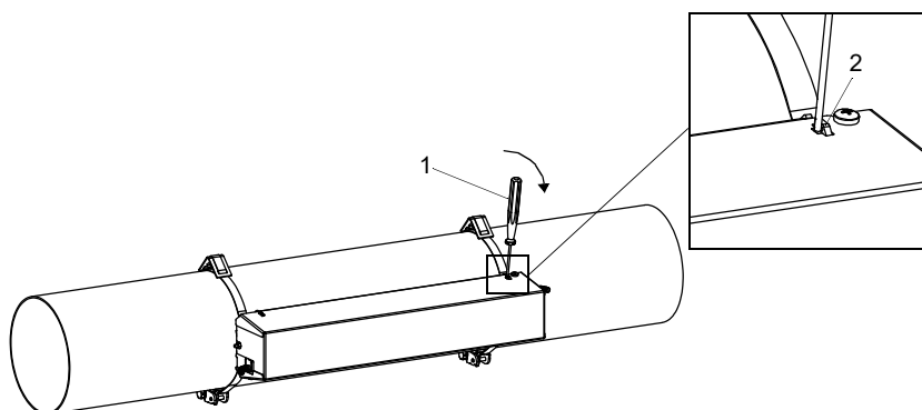
Abb. 7.59: Entfernen der Abdeckung
