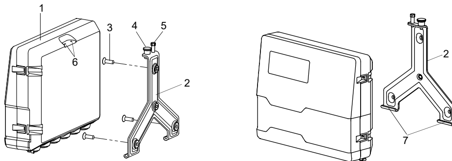
Abb. 7.5: Montageansicht
