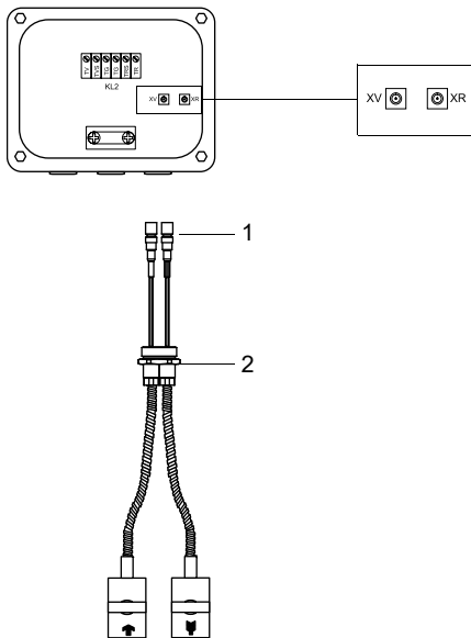
Abb. 8.6: Anschluss des Sensorkabels mit SMB-Steckern
