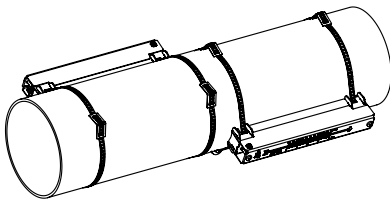
Abb. 7.11: Sensorbefestigung Variofix L (Durchstrahlungsanordnung)
