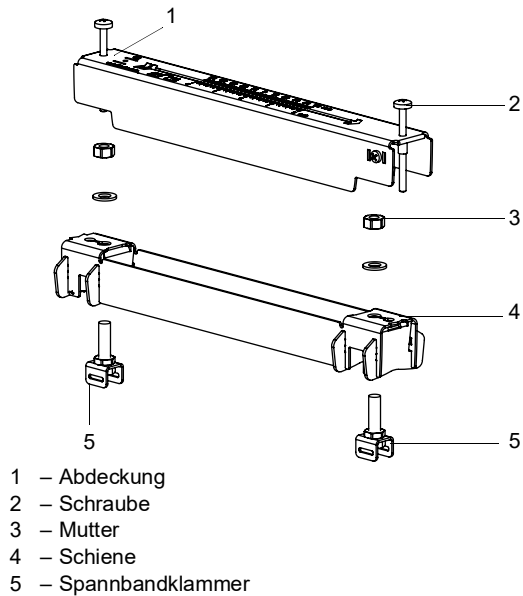
Abb. 7.13: Demontage von Variofix L
