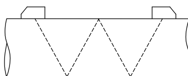
Abb. 4.5: Reflexanordnung mit 1 Strahl und 4 Schallwegen
