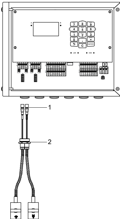
Abb. 8.2: Anschluss des Sensorkabels mit SMB-Steckern an den Messumformer
