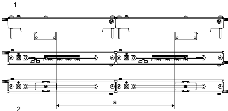
Abb. 7.32: Einstellen des Sensorabstands
