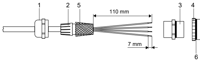
Abb. 8.21: Konfektionierung des Verlängerungskabels
