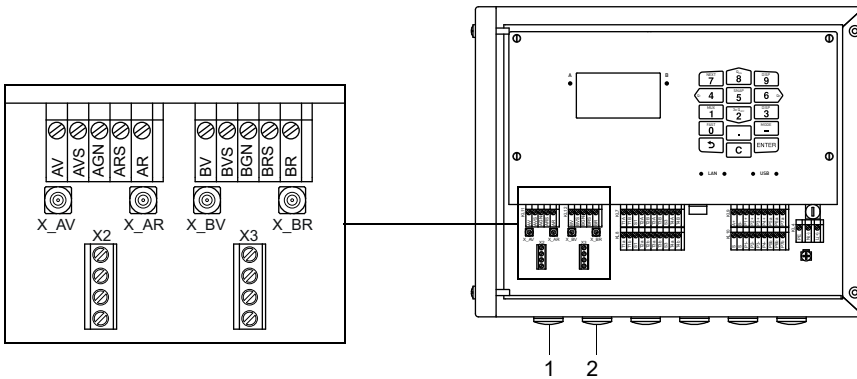
Abb. 8.1: Anschluss der Sensoren am Messumformer
