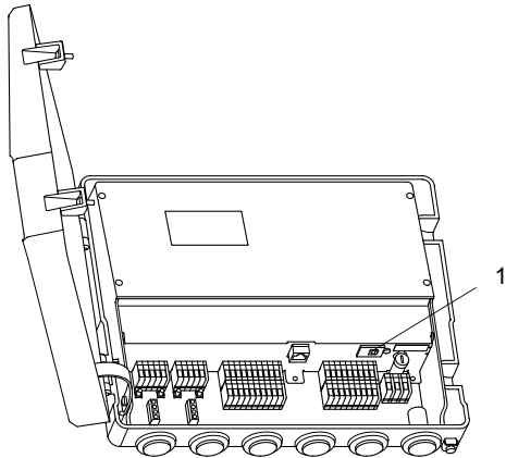
Abb. 8.23: Anschluss des USB-Kabels
