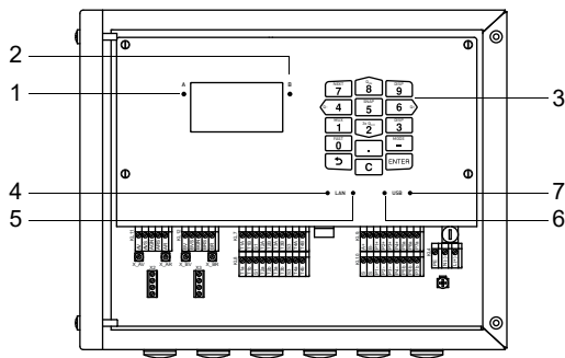
Abb. 9.1: Bedienungsfeld des Messumformers
