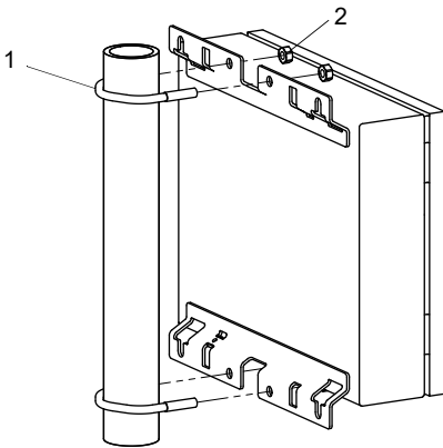
Abb. 7.6: Montageansicht
