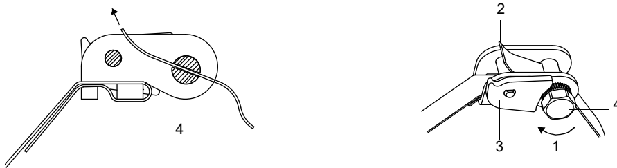
Abb. 7.54: Ratschenschloss mit Spannband
