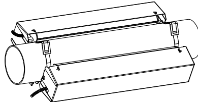
Abb. 7.36: Sensorbefestigung Variofix C (Durchstrahlungsanordnung)
