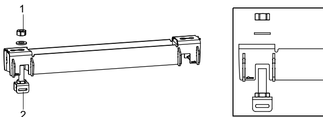
Abb. 7.23: Schiene mit Spannbandklammer
