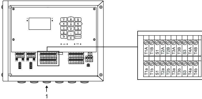
Abb. 8.18: Anschluss der Temperaturfühler am Messumformer
