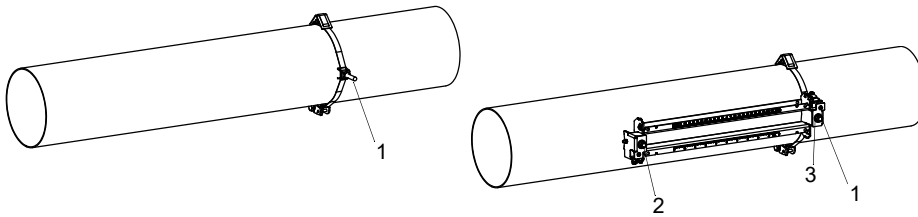
Abb. 7.49: Schiene einseitig am Rohr befestigt
