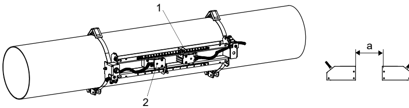
Abb. 7.55: Sensoren in Schiene (Federbügel nicht dargestellt)
