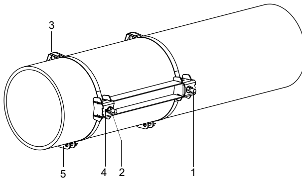
Abb. 7.25: Schiene am Rohr
