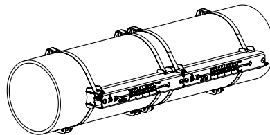
Abb. 7.12: Sensorbefestigung Variofix L (Reflexanordnung)
