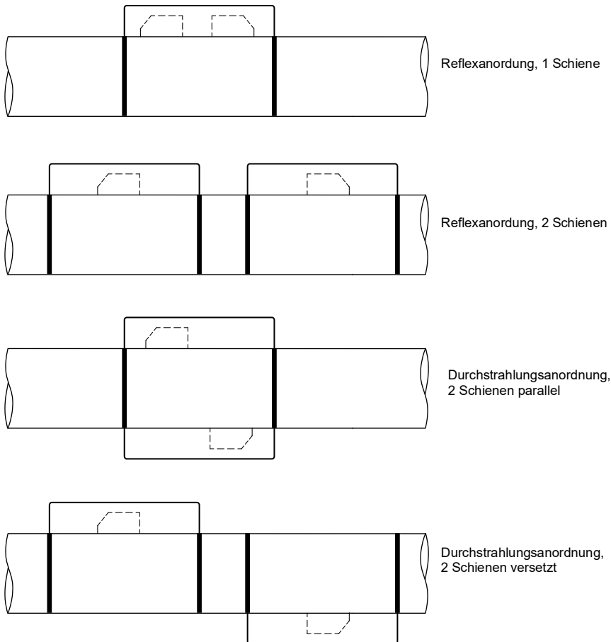
Abb. 7.9: Anordnung der Sensoren in Montage-Schienen
