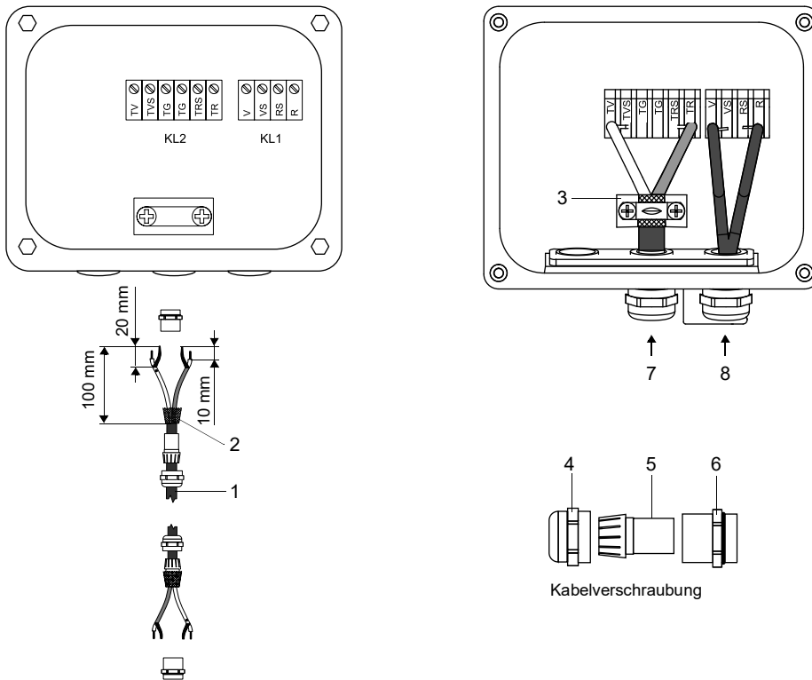
Abb. 8.10: Anschluss des Verlängerungskabels an das Klemmgehäuse (mit Potentialtrennung)
