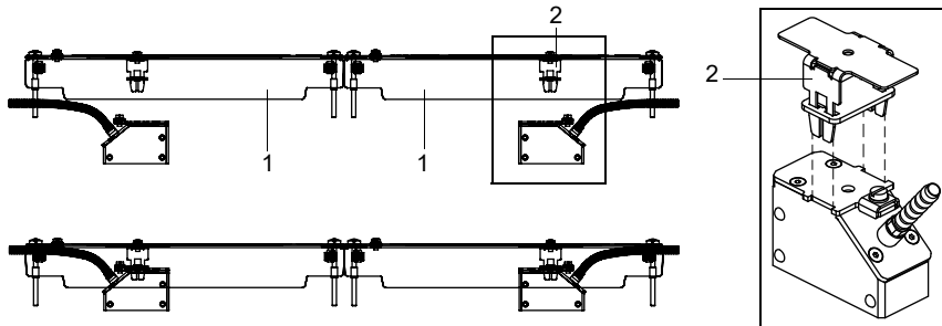
Abb. 7.31: Einbauen der Sensoren in die Abdeckungen
