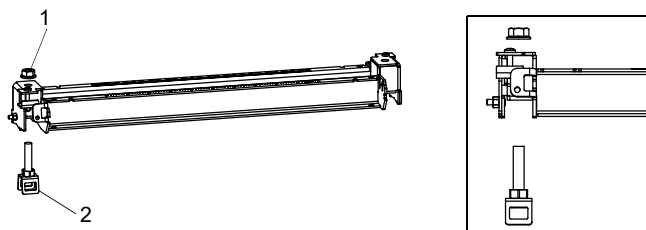
Abb. 7.48: Schiene mit Spannbandklammer
