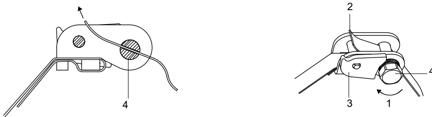
Abb. 6.22: Ratschenschloss mit Spannband
