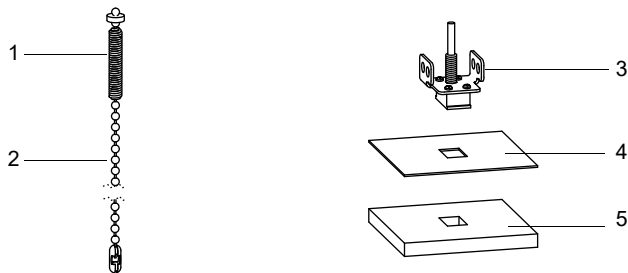
Abb. 6.65: Temperaturfühler
