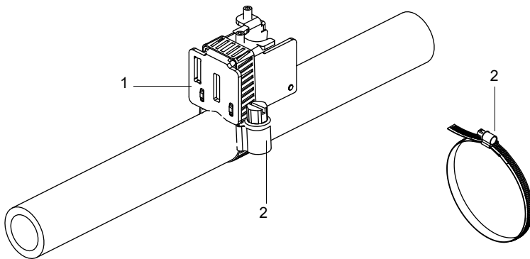
Abb. 6.60: Sensor im Montageschuh, montiert mit Spannband und Spannschloss
