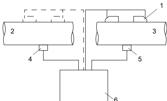
Abb. 20.1: Wärmestrommessung bei Durchflussmessung
