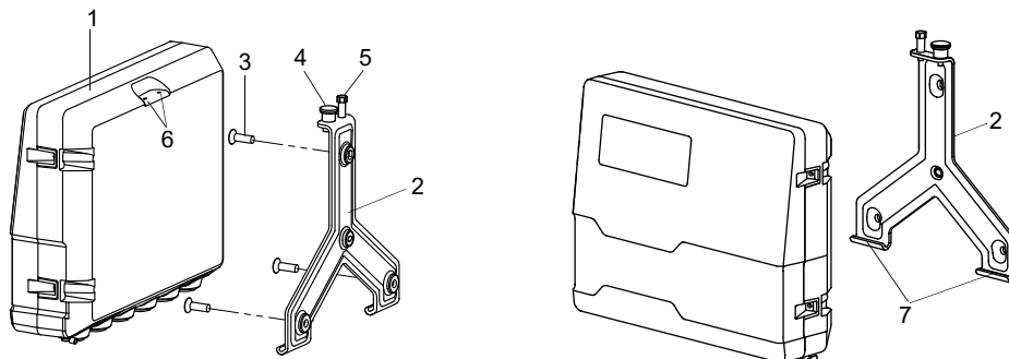
Abb. 6.5: Montageansicht
