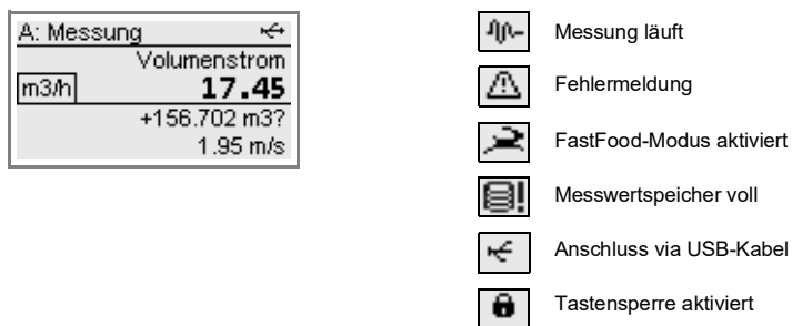
Abb. 4.4: Statusanzeigen (Zeile 1)
