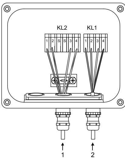
Abb. 7.22: Klemmgehäuse
