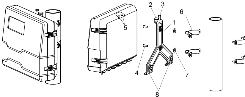
Abb. 6.7: Montageansicht
