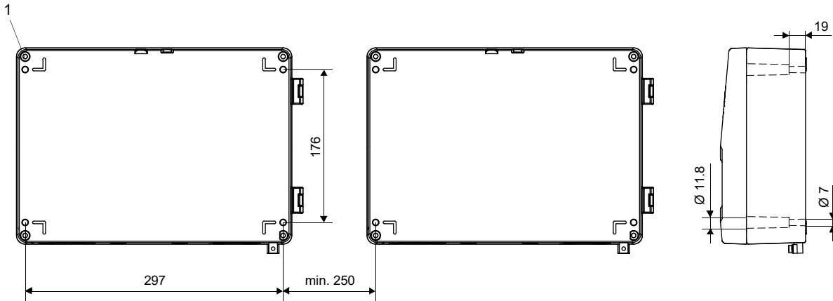
Abb. 6.4: Messumformer (Abmessungen in mm)
