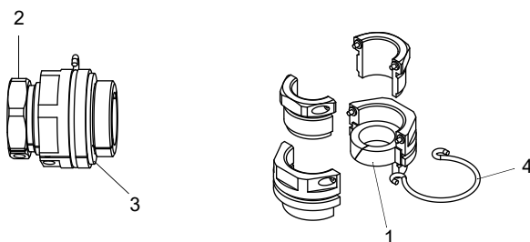
Abb. 7.18: Split-Kabelverschraubung
