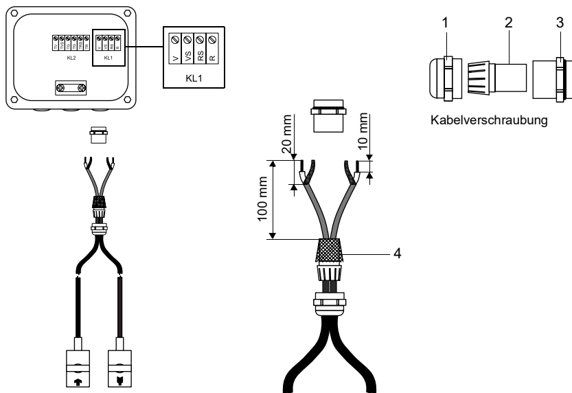
Abb. 7.7: Anschluss des Sensorkabels mit Kunststoffkabelmantel und abisolierten Kabelenden
