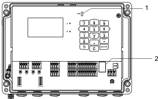
Abb. 7.17: Serviceschnittstellen am Messumformer
