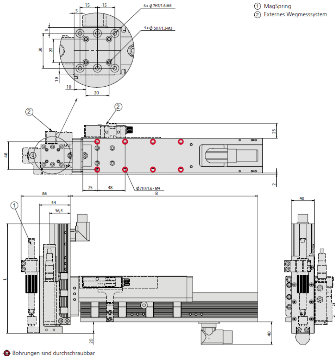
Abb. 2 Maßzeichnung EPS midi YZ
