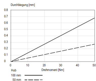
Durchbiegung ES20-SL
