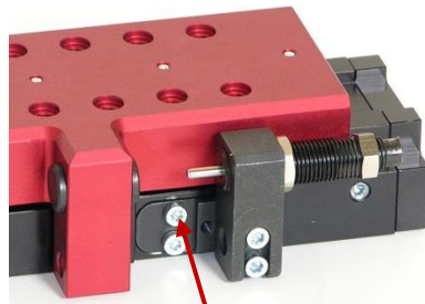
Abb. 19 Hub-Reduzierung (normal)
