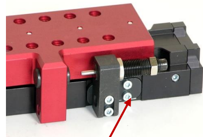
Reduzierter Hub
