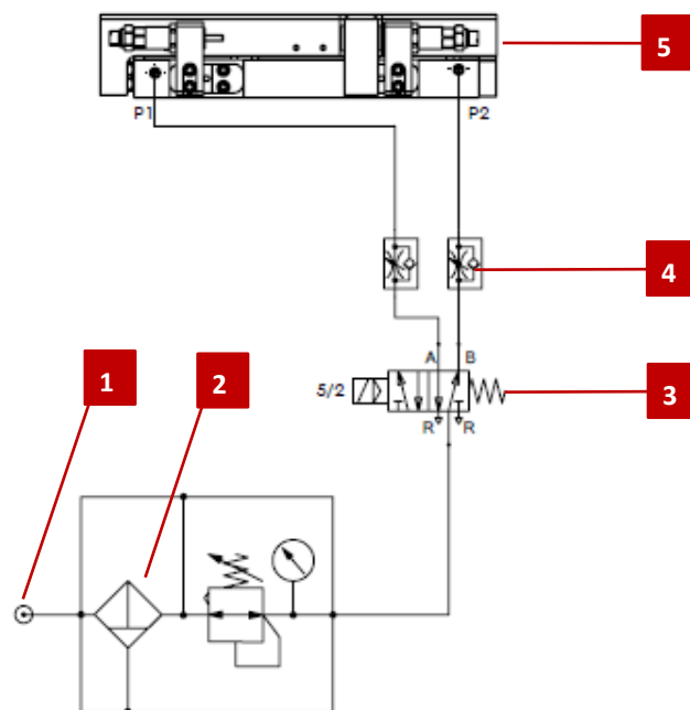
Abb. 10 Pneumatik-Schaltplan Compact-Schlitten
