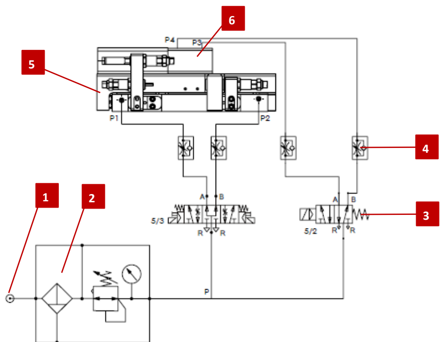
Abb. 10 Pneumatik-Schaltplan Compact-Schlitten
