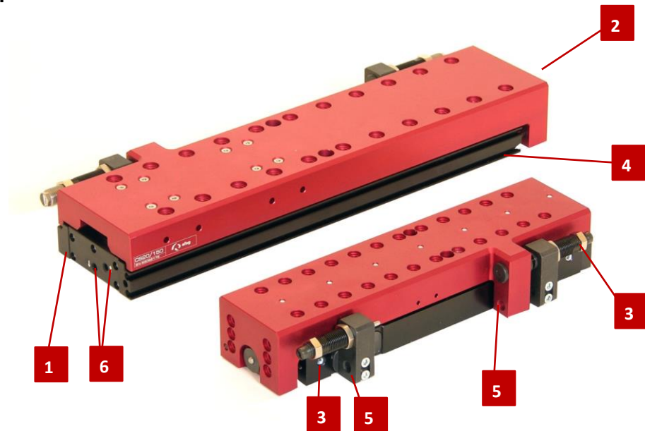
Abb. 8 Aufbau des CS Moduls
