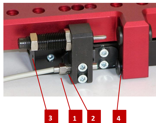
Abb. 13 Montage Induktiv-Initiator
