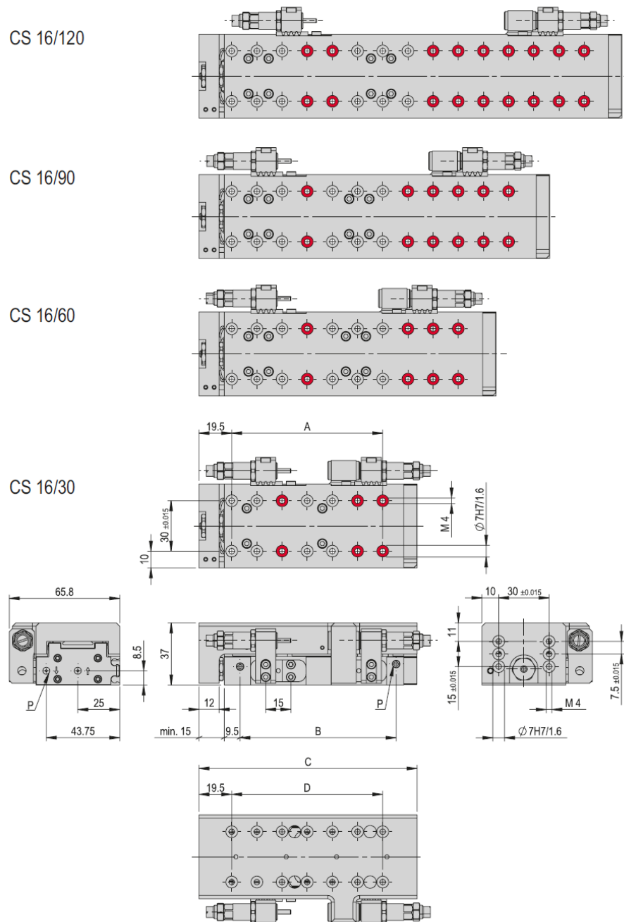
Abb. 1 Masszeichnung Compact-Schlitten CS 16
