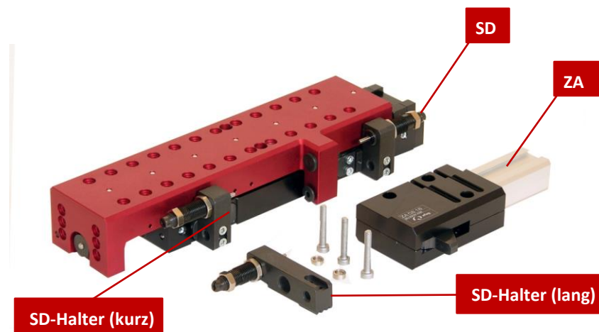
Abb. 21 ZA-Zwischenanschlag montieren
