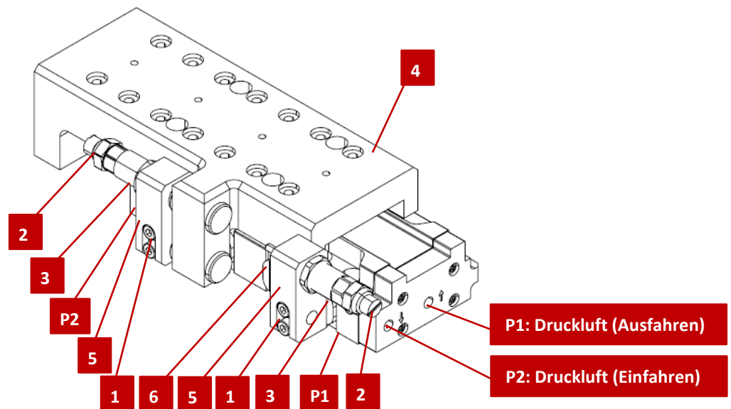
Abb. 26 Einbau und Einstellung Compact-Schlitten
