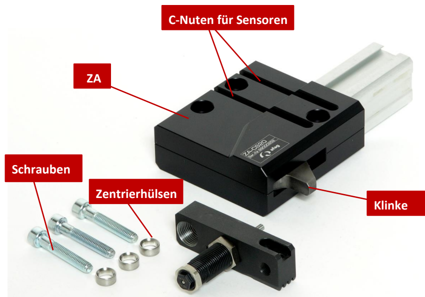
Abb. 20 Übersicht des ZA-Zwischenanschlags
