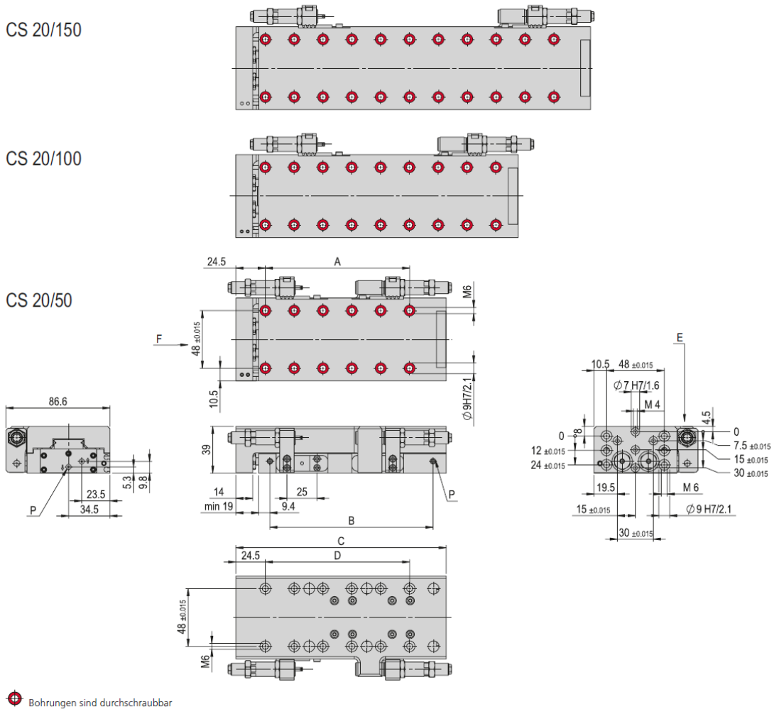
Abb. 4 Masszeichnung Compact-Schlitten CS 20
