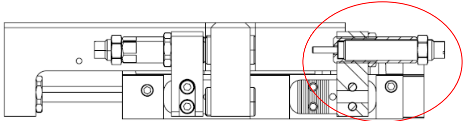
Abb. 15 Maximale Dämpferwirkung
