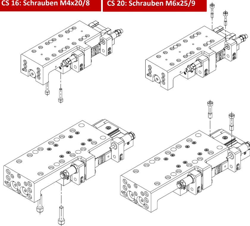
Abb. 9 Montage Grundkörper von unten Montage Grundkörper von oben
