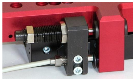
Abb. 18 Sensor (einstellbar)
