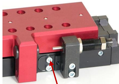
Abb. 19 Hub-Reduzierung (normal)
