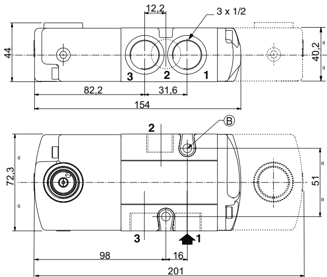
TYPE 01 : Surmoulée époxy SC : CEI 335 / ISO 4400
