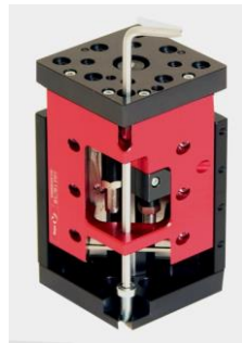
Abb. 8 Durchschraubbare Hubmodule
