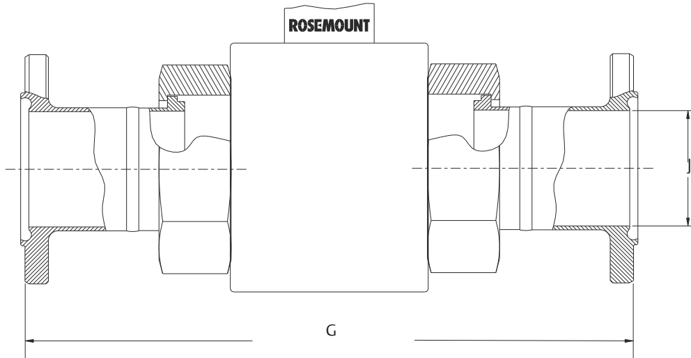
그림 32: 8721 위생용 센서 SMS1145
