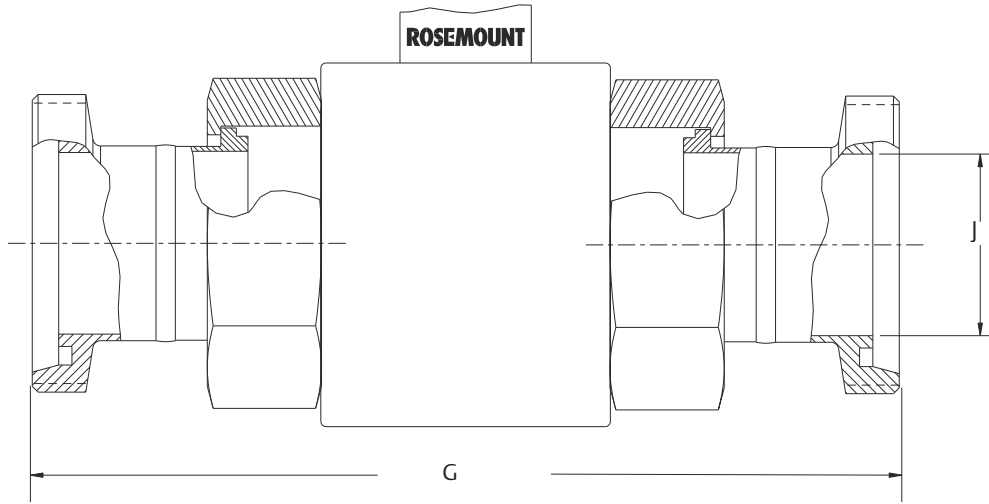
그림 29: 8721 위생용 센서 DIN 11851(미터식)
