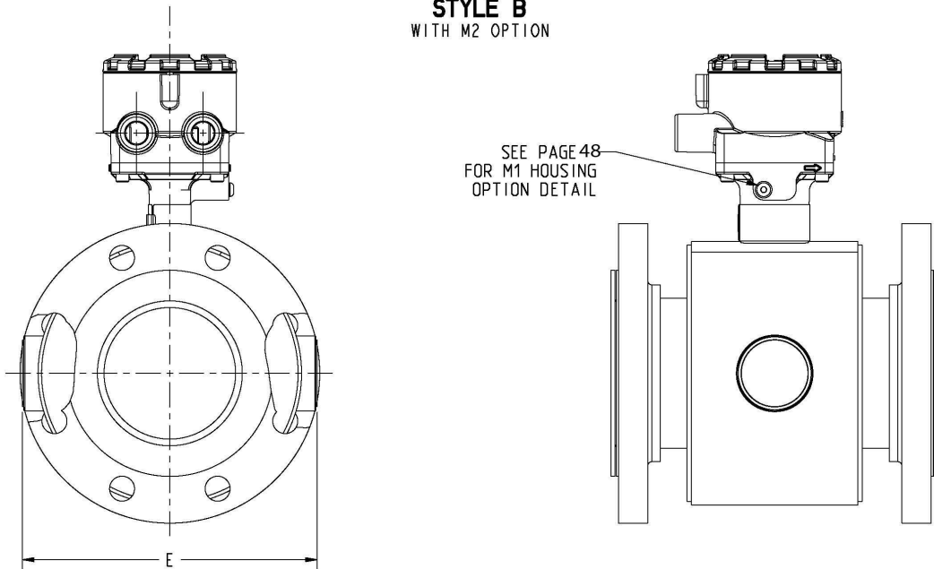
그림 17: 8705-M 플랜지 센서 1/2인치~36인치 (DN 15mm~900mm) M2/M4 코일 하우징(P ≤ Class 600 감소)
