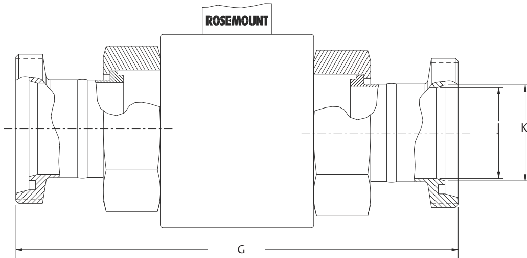
그림 30: 8721 위생용 센서 DIN 11864-1
