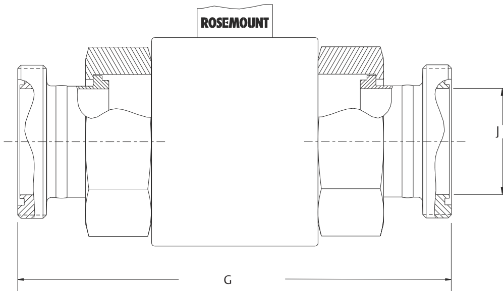
그림 32: 8721 위생용 센서 SMS1145
