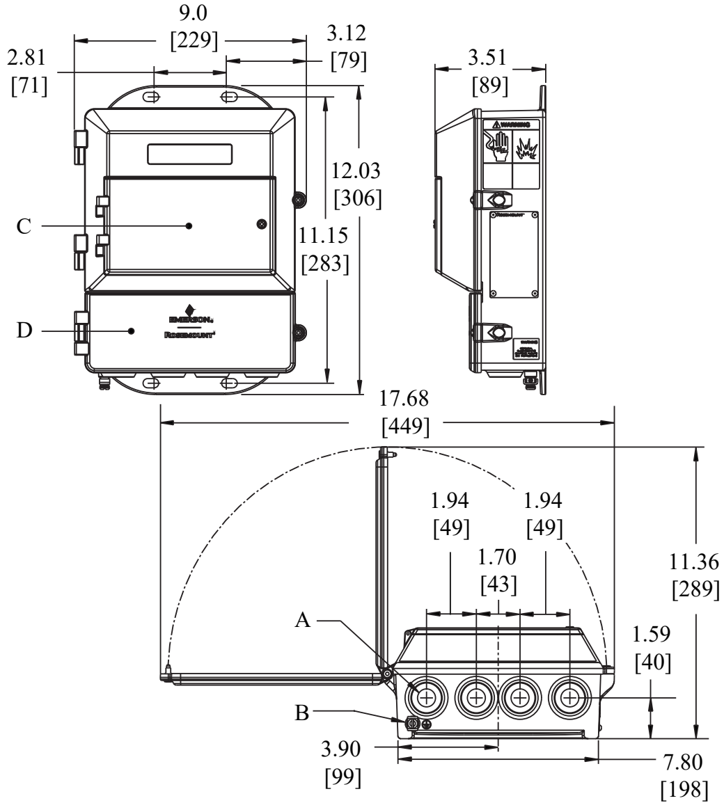
그림 12: 8712 벽면 설치 트랜스미터 치수
