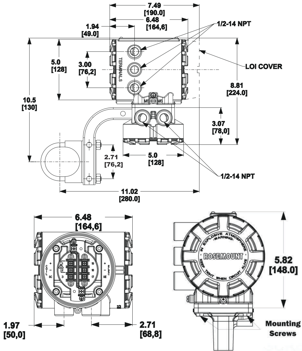
그림 13: 8732 현장 설치 트랜스미터 치수
