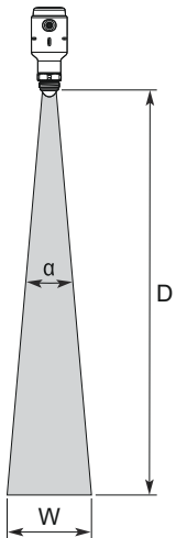
그림 11: 빔 각도 및 빔 너비
