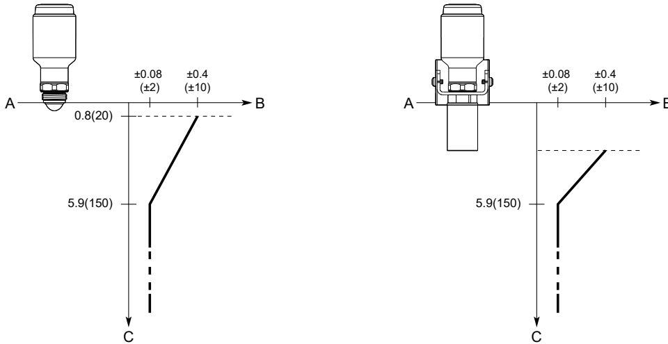
그림 4: 측정 범위 정확도
