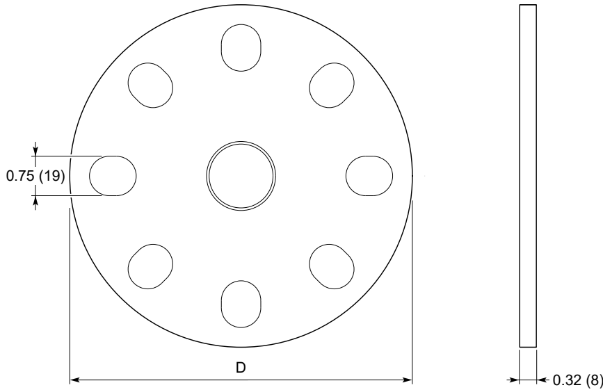
그림 15: 비가압 어플리케이션 플랜지
