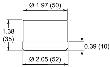
그림 17: D50 용접 어댑터
