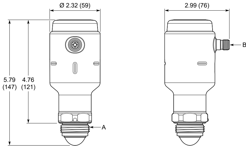
그림 14: Rosemount 1408A
