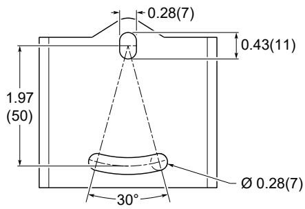
그림 19: 구멍 패턴
