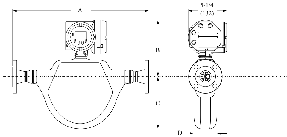
그림 2: CMFS 025, 040, 050, 075, 100 및 150
