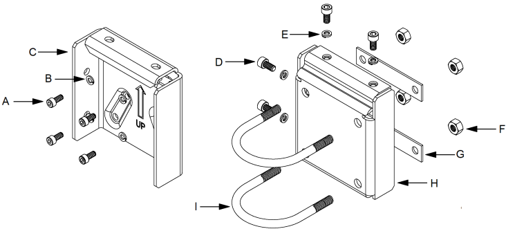
그림 4-3: 마운팅 브라켓 키트 구성품
