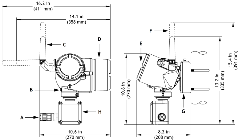
그림 6-1: Rosemount 4390 무선 트랜스미터 치수
