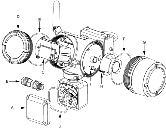
그림 5-2: 예비 부품 개요
