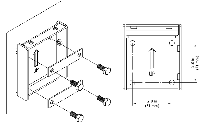
그림 4-5: 벽면 및 랙 장착
