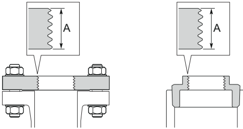
그림 3-1: 나사산 결합 길이
