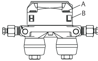
그림 1-5: 적절한 볼트 설치
