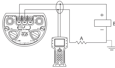
그림 4-3: 트랜스미터 배선(정선박스 하우징)
