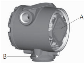
그림 3-1: 트랜스미터 하우징 고정 나사
