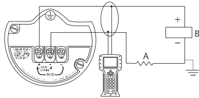
그림 4-2: 트랜스미터 배선(Plantweb 하우징)
