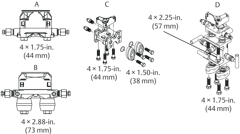
그림 1-4: 일반적인 트랜스미터 어셈블리
