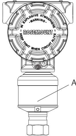
그림 1-6: 인라인 게이지 트랜스미터
