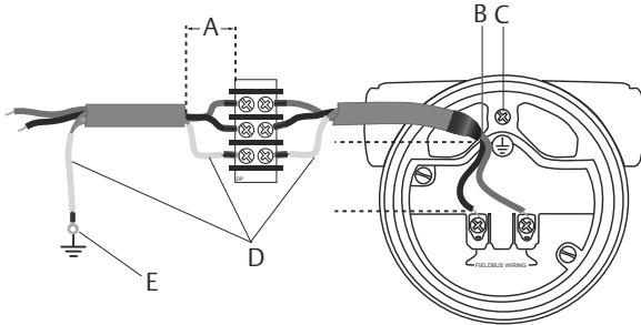
그림 4-1: 트랜스미터 배선
