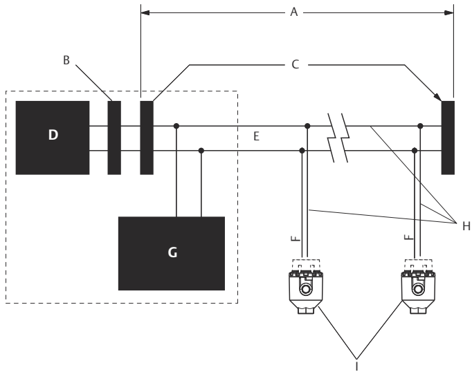
그림 3-2: Fieldbus Networking에 대한 일반 구성
