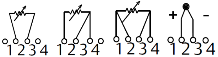
그림 3-1: 센서 연결
