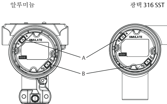
그림 2-4: 트랜스미터 전자 장치 보드
