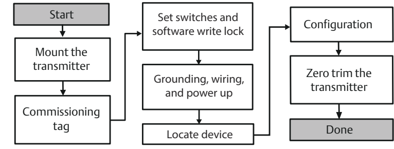
그림 2-1: 설치 순서도
