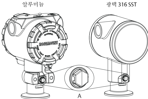
그림 2-2: 인라인 보호 게이지 벤트 아래쪽 압력 포트
