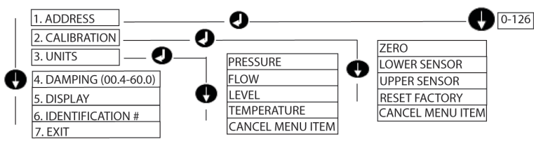
그림 3-1: LOI 메뉴
