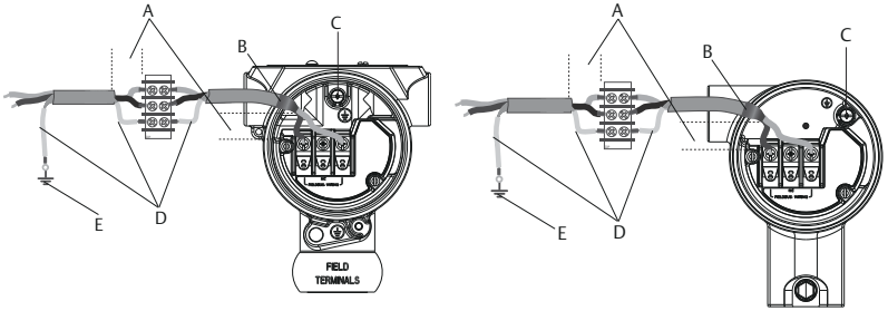
그림 2-5: 배선
