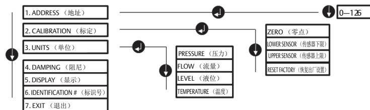
图 8. LOI 菜单
