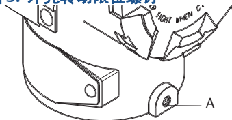
A. 外壳转动限位螺钉（ 5/64 英寸）
