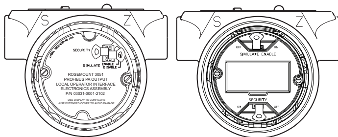
图 4. 变送器跳线位置
