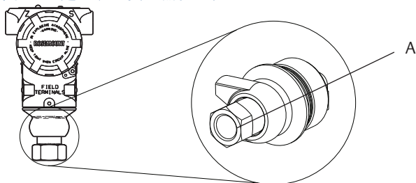
A. 低压侧端口（大气压力参考）
