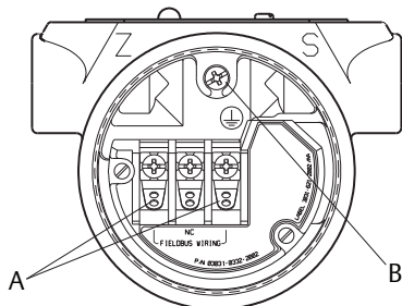
图 5. 端子
