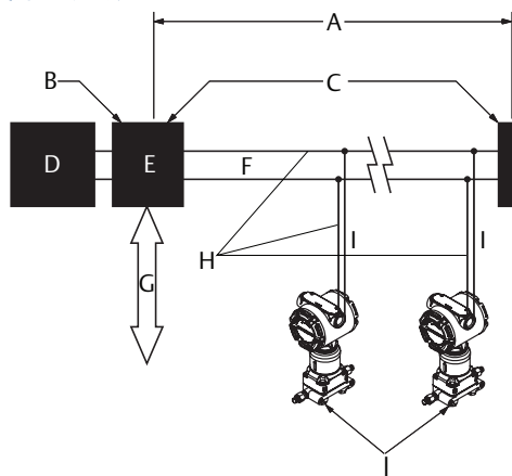
图 6. 接线
