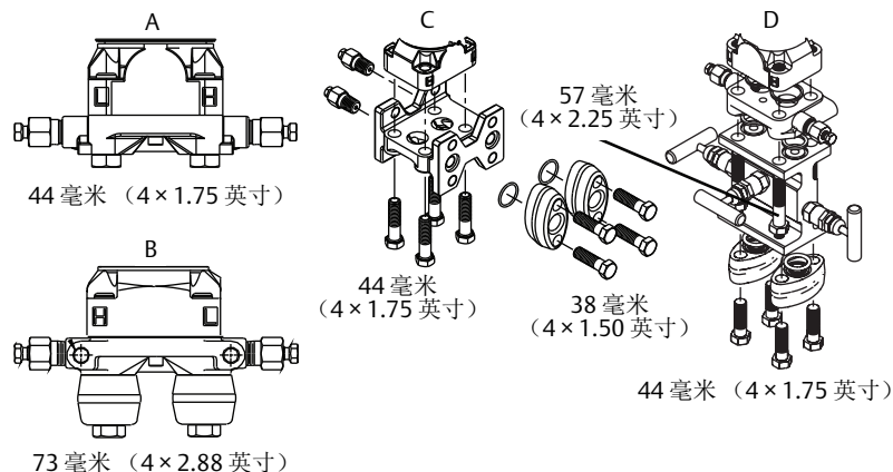
图 1. 常用变送器组件
