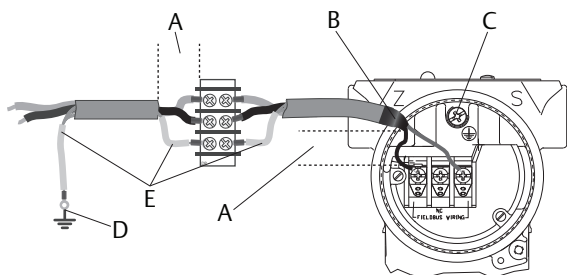
图 7. 接线
