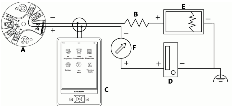
図 2-1: ベンチループへのフィールドコミュニケーターの接続
