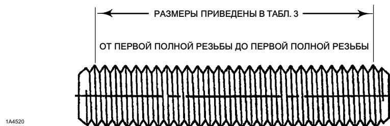
Рис. 2. Длина шпильки фланца для соединения предохранителя уплотнения
