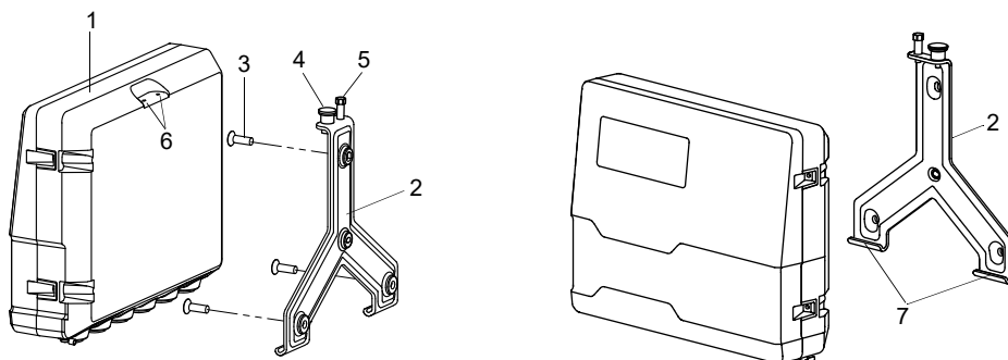
Рис. 7.5: Вид установки
