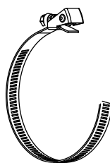
Рис. 7.15: Быстросъемный замок со стальной лентой
