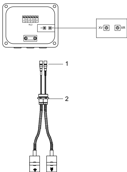
Рис. 8.6: Подключение кабеля датчика со штекерами SMB
