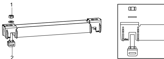
Рис. 7.23: Рельс с зажимом для стальной ленты
