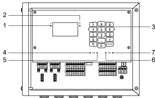
Рис. 9.1: Панель управления преобразователя
