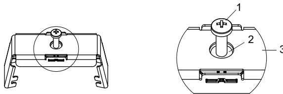
Рис. 7.56: Пружинная скоба
