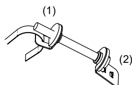
Рис. 7.62: Замок FLEXIM
