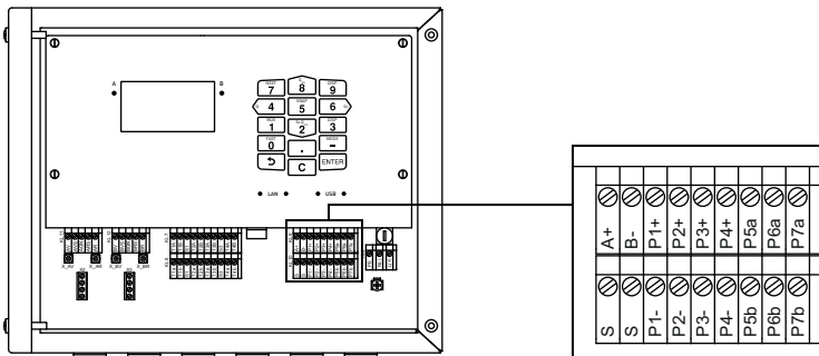
Рис. 8.16: Подключение выходов к преобразователю
