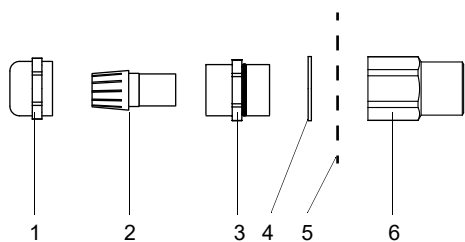
Рис. 7.22: Кабельный сальник
