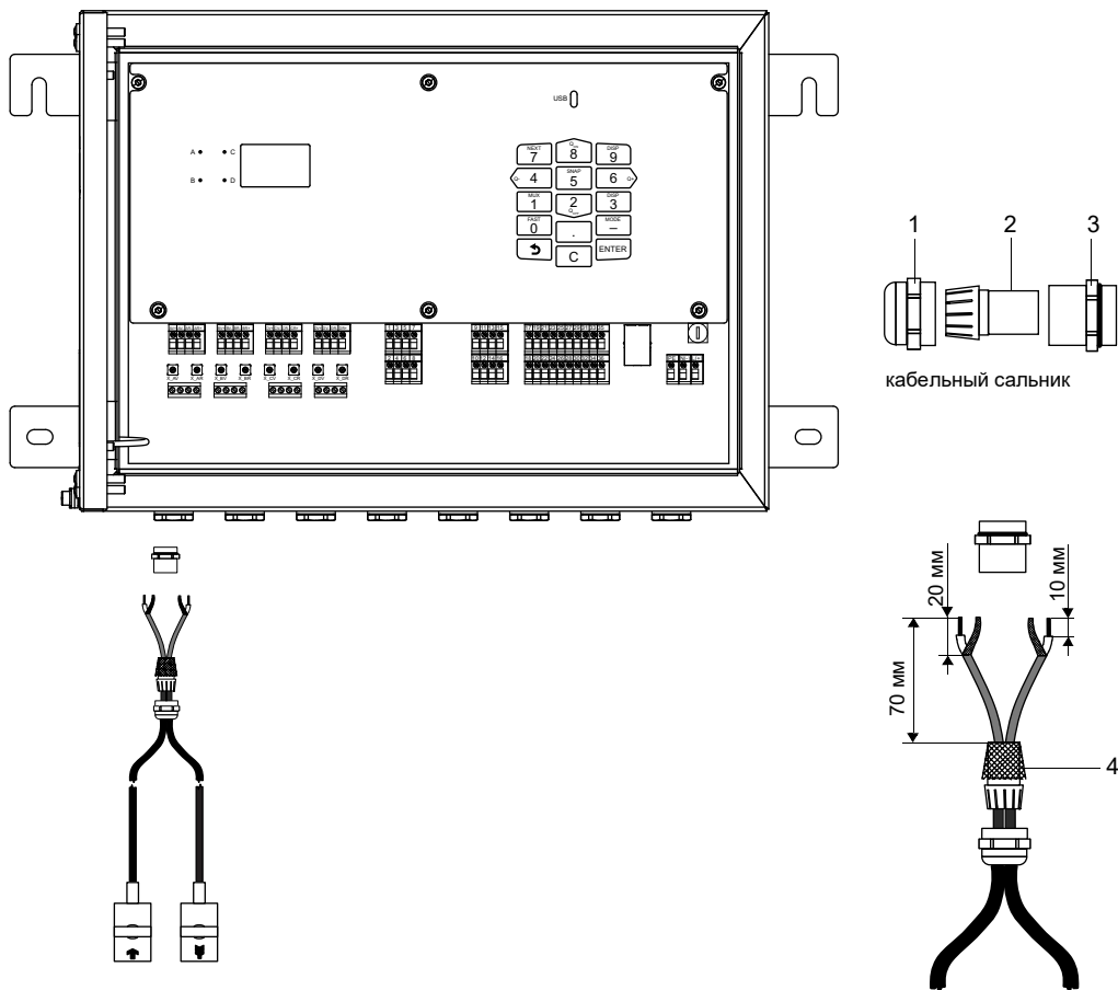
Рис. 7.3: Подключение кабеля датчика с пластмассовой изоляцией и неизолированными концами к преобразователю
