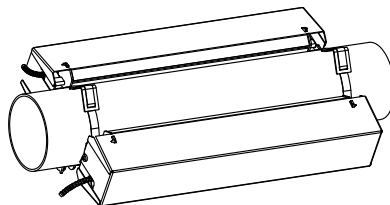
Рис. 6.33: Крепление датчика Variofix C (режим диагональ)
