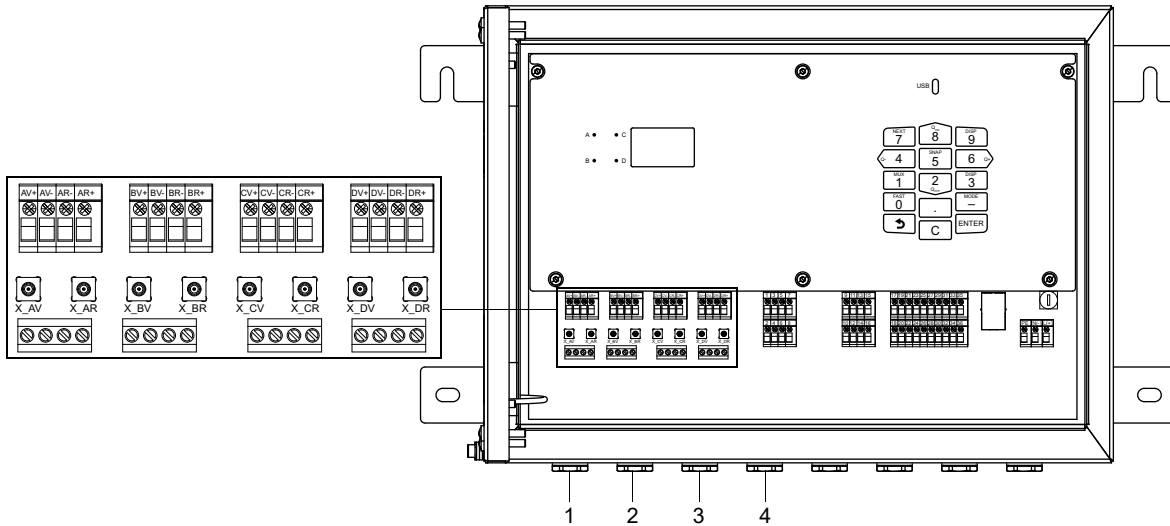
Рис. 7.1: Подключение датчиков к преобразователю
