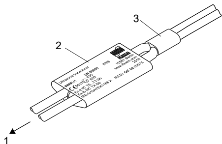
Рис. 6.7: Фабричная табличка на кабеле датчика
