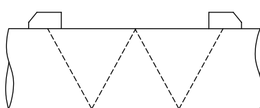
Рис. 3.6: Режим отражения с 1-м лучом и 4-мя проходами звука
