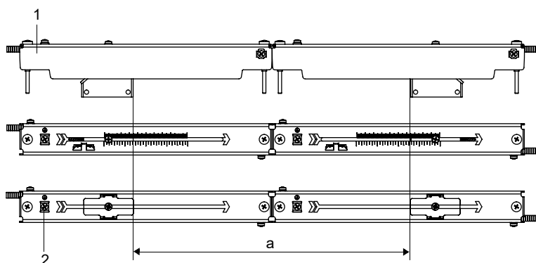
Рис. 6.29: Установка расстояния между датчиками
