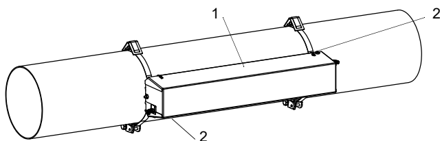
Рис. 6.55: Крепление Variofix C с датчиками на трубе
