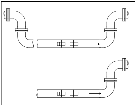
Рис. 3.13: Рекомендуемое размещение датчиков
