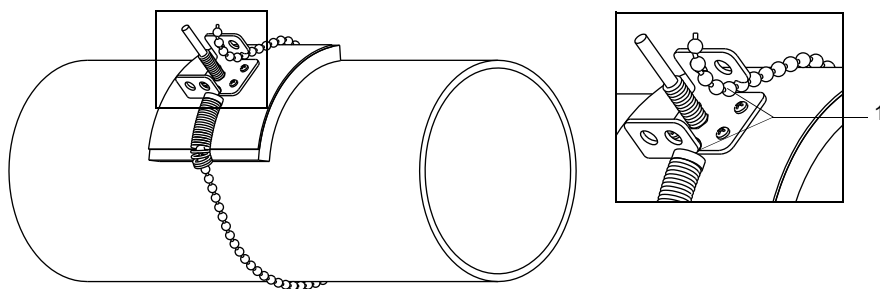
Рис. 6.63: Датчик температуры на трубе
