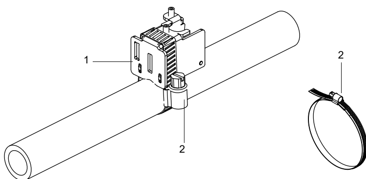
Рис. 6.57: Датчик в монтажном башмаке, установленный с помощью стальной ленты и замка
