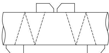
Рис. 3.5: Режим диагональ с 2-мя лучами и 3-мя проходами звука
