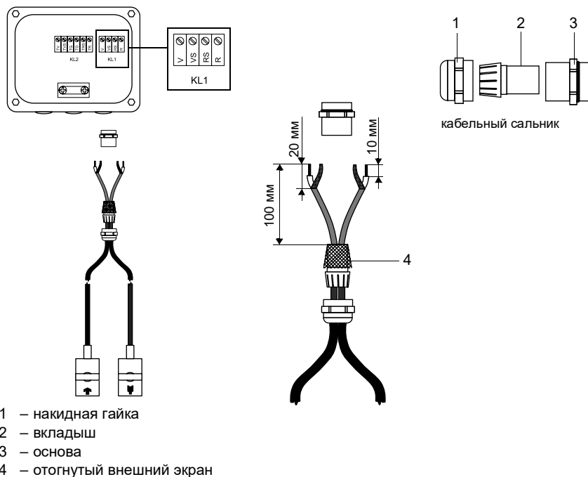
Рис. 7.7: Подключение кабеля датчика с пластмассовой изоляцией и неизолированными концами
