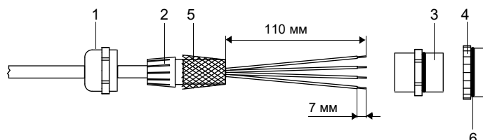
Рис. 7.18: Разделка удлинительного кабеля
