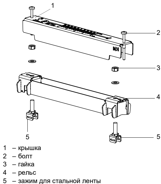
Рис. 6.10: Разборка крепления датчика Variofix L
