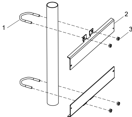
Рис. 6.3: Установка крепежной пластины для прибора
