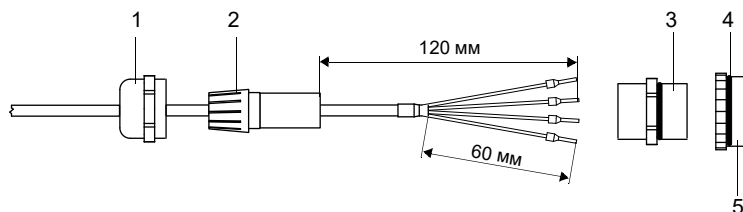
Рис. 7.17: Разделка датчика температуры
