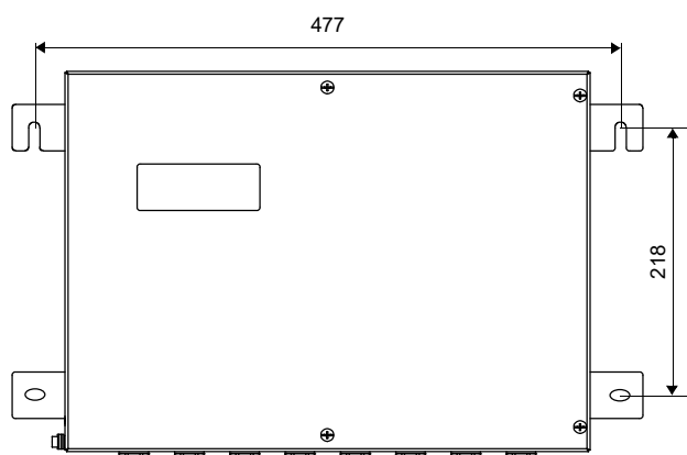
Рис. 6.2: Преобразователь (размеры в мм)
