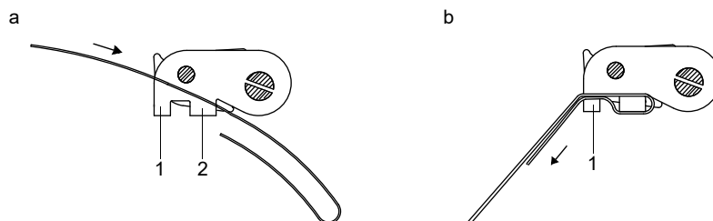
Рис. 6.38: Храповой замок со стальной лентой
