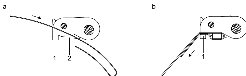
Рис. 6.13: Храповой замок со стальной лентой
