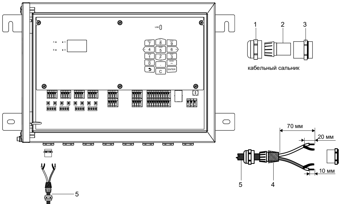
Рис. 7.5: Подключение удлинительного кабеля к преобразователю
