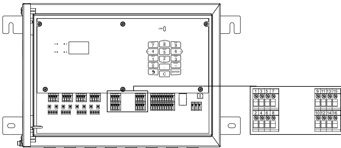
Рис. 7.15: Подключение входов к преобразователю
