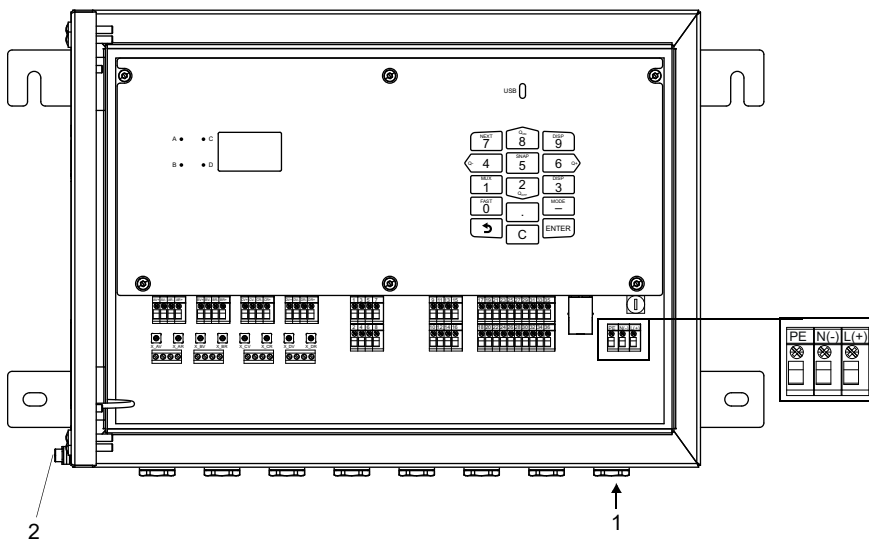
Рис. 7.12: Подключение питания напряжения к преобразователю
