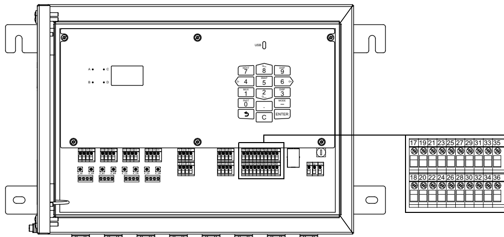
Рис. 7.14: Подключение выходов к преобразователю
