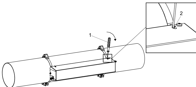
Рис. 6.56: Снятие крышки
