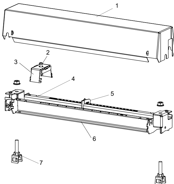
Рис. 6.35: Разборка крепления датчика Variofix C
