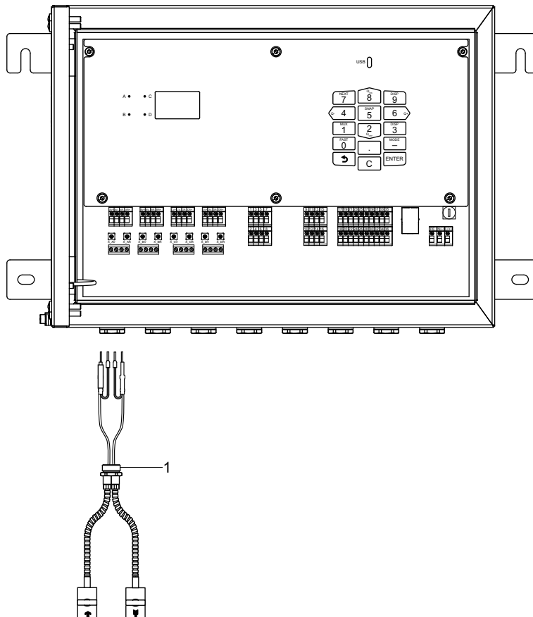
Рис. 7.4: Подключение кабеля датчика с кабелепроводом из нержавеющей стали и неизолированными концами к преобразователю
