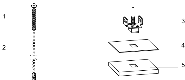
Рис. 6.62: Датчик температуры
