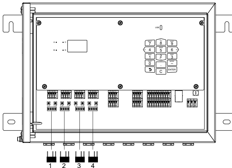
Рис. 7.11: Память SENSPROM
