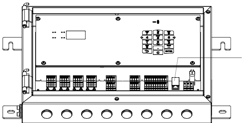
Рис. 7.21: Подключение кабеля ЛВС
