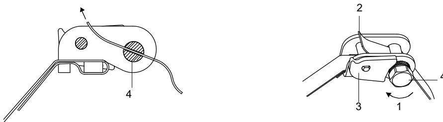
Рис. 6.51: Храповой замок со стальной лентой
