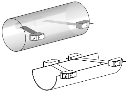
Рис. 3.7: 2 луча в одной плоскости
