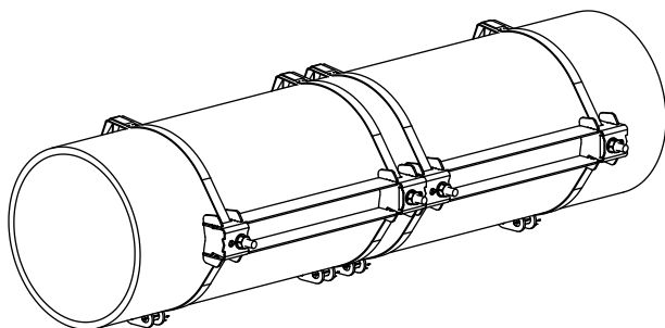
Рис. 6.27: Труба с 2-мя рельсами
