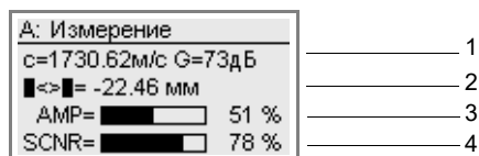
Рис. 9.1: Индикация диагностики
