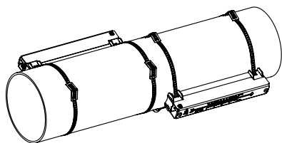
Рис. 6.8: Крепление датчика Variofix L (режим диагональ)
