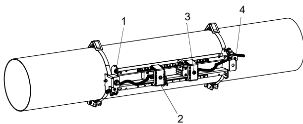
Рис. 6.54: Датчики на рельсе
