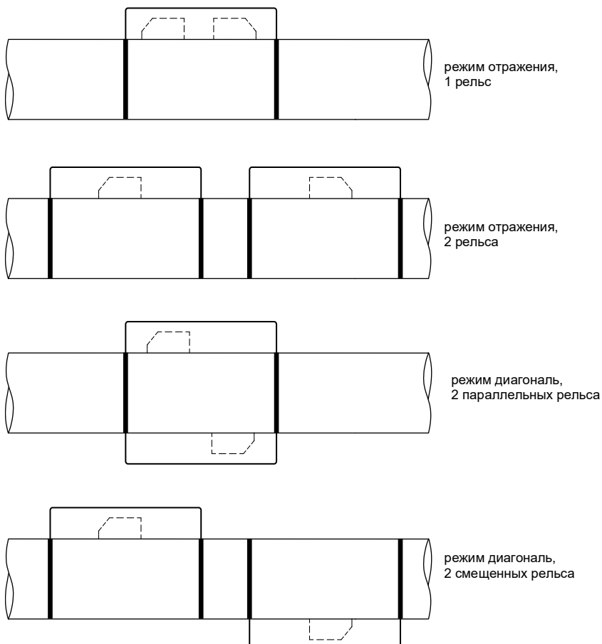
Рис. 6.6: Размещение датчиков в монтажных рельсах
