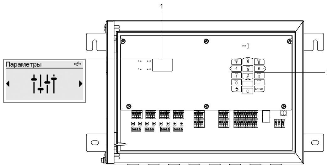
Рис. 4.2: Панель управления преобразователя
