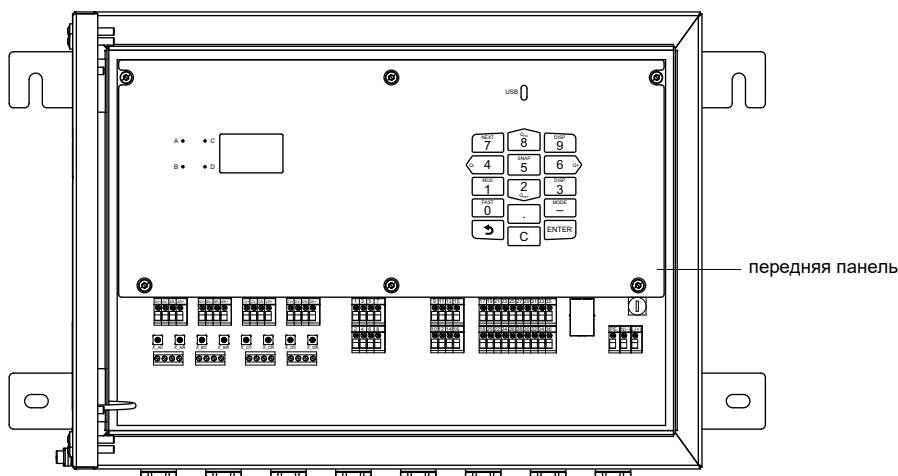
Рис. 2.1: Преобразователь
