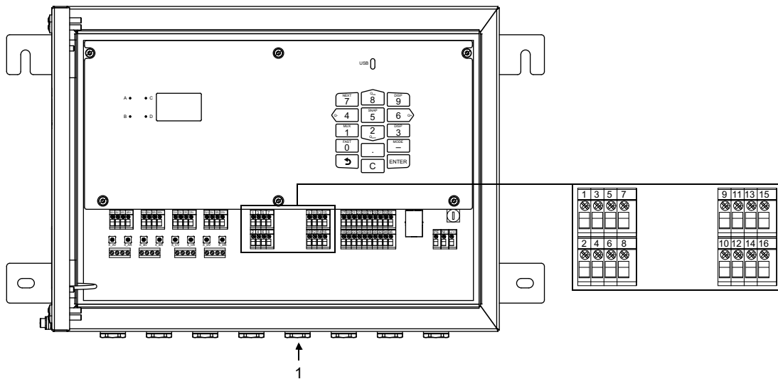
Рис. 7.16: Подключение датчиков температуры к преобразователю
