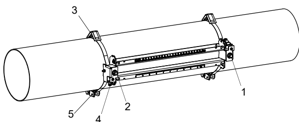
Рис. 6.47: Рельс на трубе
