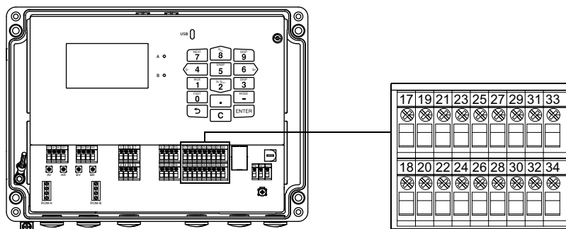
Рис. 7.15: Подключение выходов к преобразователю
