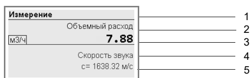
Рис. 9.2: Индикация измеряемых значений
