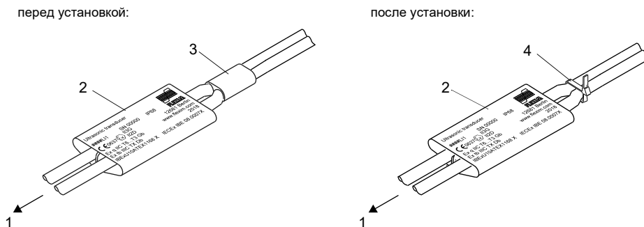
Рис. 6.9: Фабричная табличка на кабеле датчика
