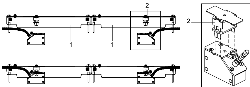
Рис. 6.30: Установка датчиков в крышки
