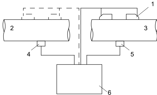
Рис. 20.1: Измерение теплового потока при измерении расхода
