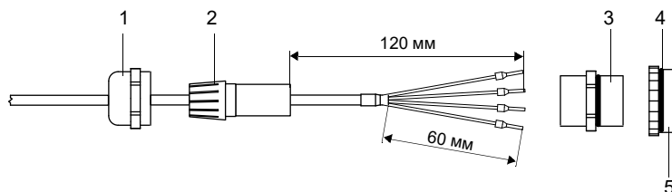
Рис. 7.18: Разделка датчика температуры
