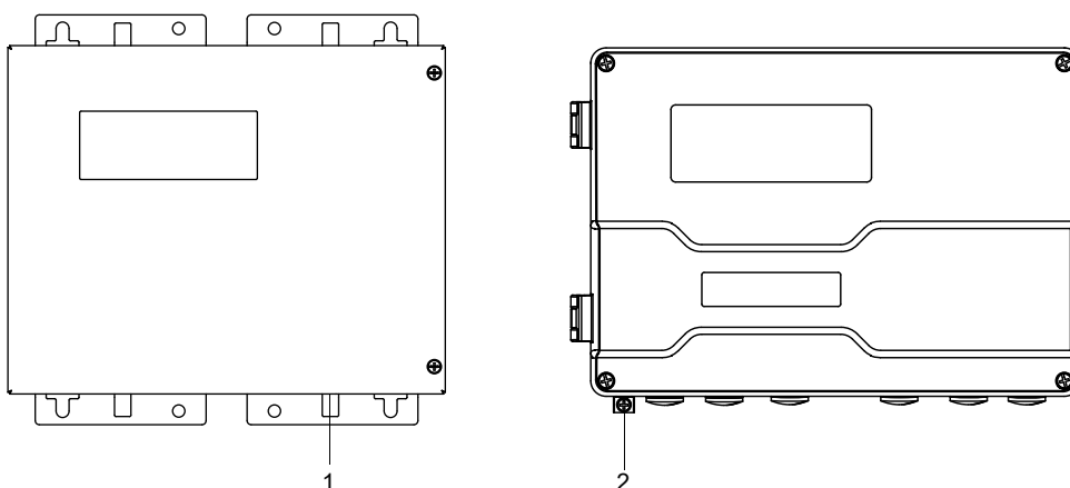
Рис. 7.12: Клемма уравнивания потенциалов на преобразователе
