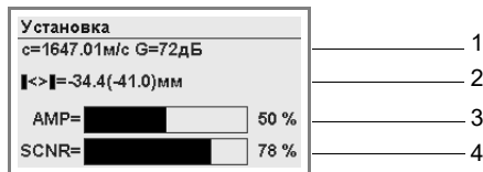
Рис. 9.1: Индикация диагностики
