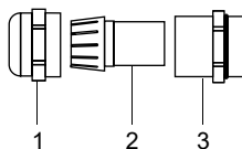
Рис. 7.14: Кабельный сальник для корпуса из алюминия
