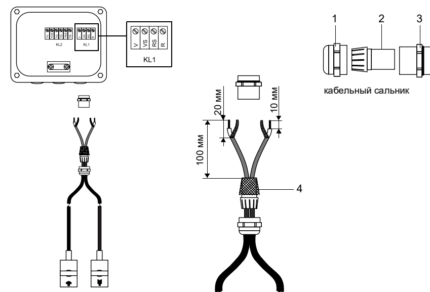
Рис. 7.7: Подключение кабеля датчика с пластмассовой изоляцией и неизолированными концами
