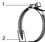
Рис. 6.26: Стальная лента с быстросъемным замком и металлической пружиной
