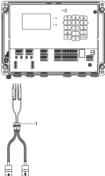
Рис. 7.4: Подключение кабеля датчика с кабелепроводом из нержавеющей стали и неизолированными концами к преобразователю
