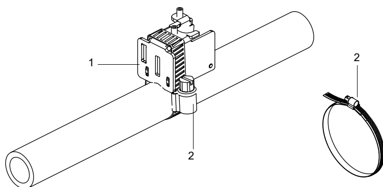
Рис. 6.59: Датчик в монтажном башмаке, установленный с помощью стальной ленты и замка
