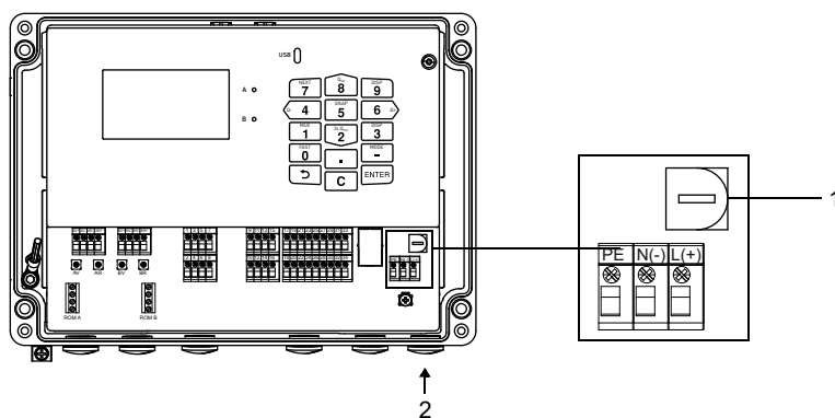
Рис. 7.13: Подключение питания напряжения к преобразователю
