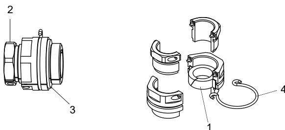
Рис. 7.22: Разъемный кабельный сальник
