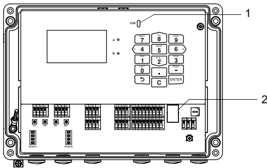
Рис. 7.21: Сервисные интерфейсы на преобразователе
