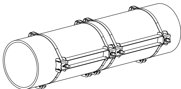
Рис. 6.30: Труба с 2-мя рельсами
