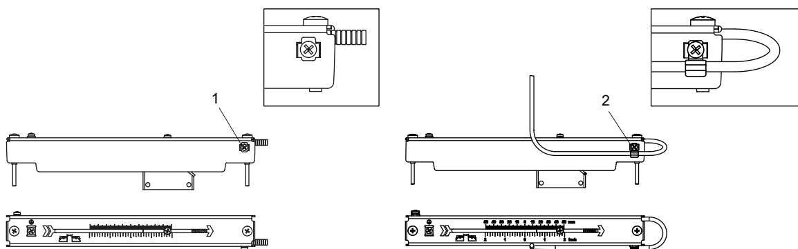
Рис. 6.33: Фиксирование кабелей датчиков
