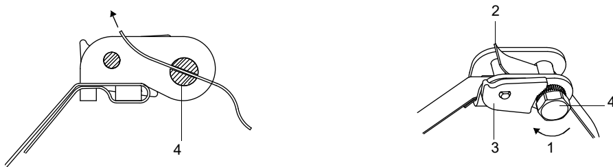
Рис. 6.47: Храповой замок со стальной лентой
