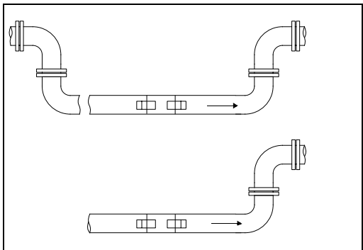
Рис. 3.14: Рекомендуемое размещение датчиков
