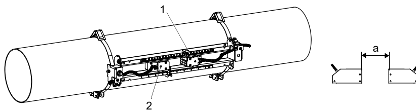
Рис. 6.55: Датчики на рельсе (пружинные скобы не изображены)
