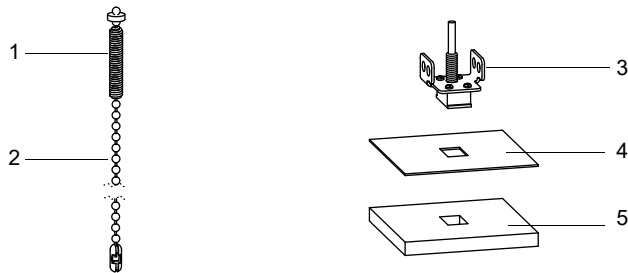
Рис. 6.65: Датчик температуры
