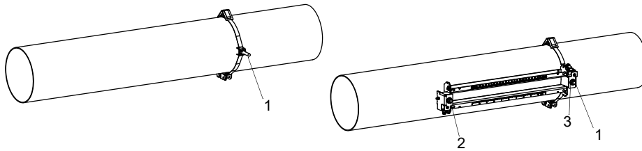
Рис. 6.49: Рельс, с одной стороны прикрепленный к трубе
