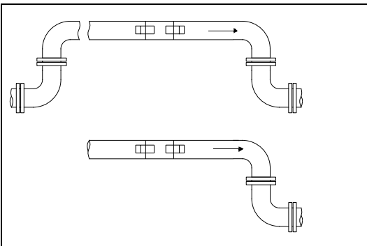
Рис. 3.15: Непригодное размещение датчиков
