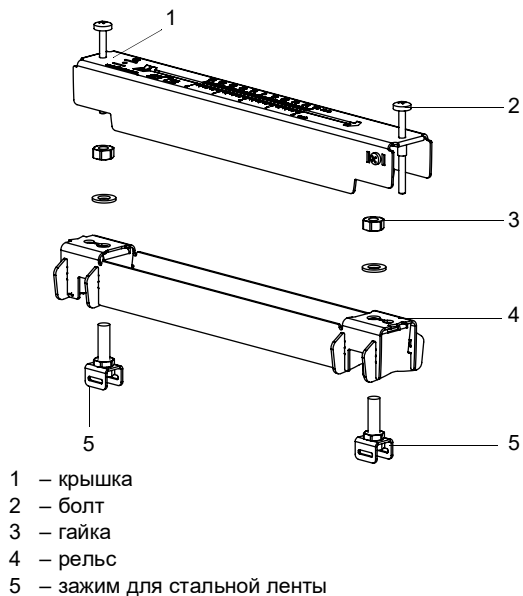
Рис. 6.13: Разборка крепления датчика Variofix L
