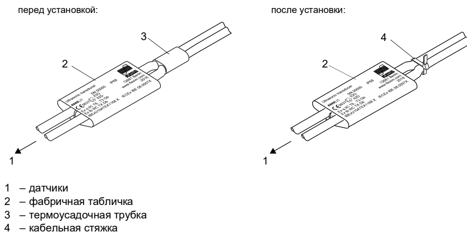
Рис. 6.10: Фабричная табличка на кабеле датчика
