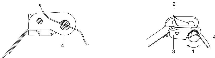
Рис. 6.54: Храповой замок со стальной лентой
