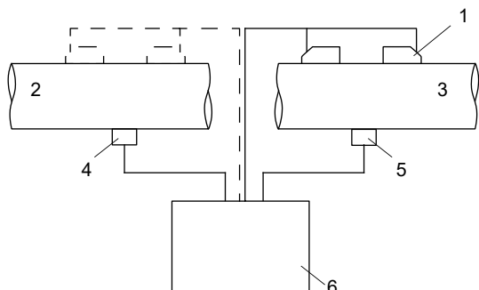
Рис. 20.1: Измерение теплового потока при измерении расхода
