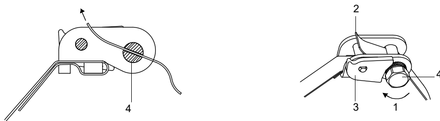
Рис. 6.22: Храповой замок со стальной лентой
