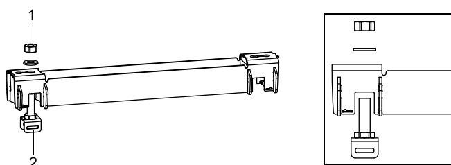
Рис. 6.23: Рельс с зажимом для стальной ленты
