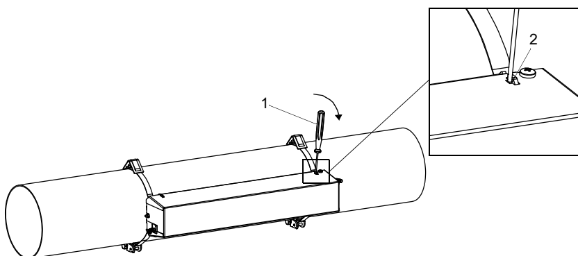
Рис. 6.59: Снятие крышки
