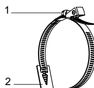
Рис. 6.52: Стальная лента с быстросъемным замком и металлической пружиной
