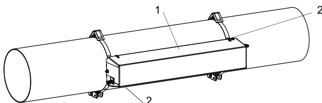
Рис. 6.58: Крепление Variofix C с датчиками на трубе
