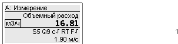
Рис. 9.3: Строка состояния
