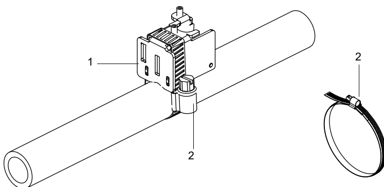
Рис. 6.60: Датчик в монтажном башмаке, установленный с помощью стальной ленты и замка
