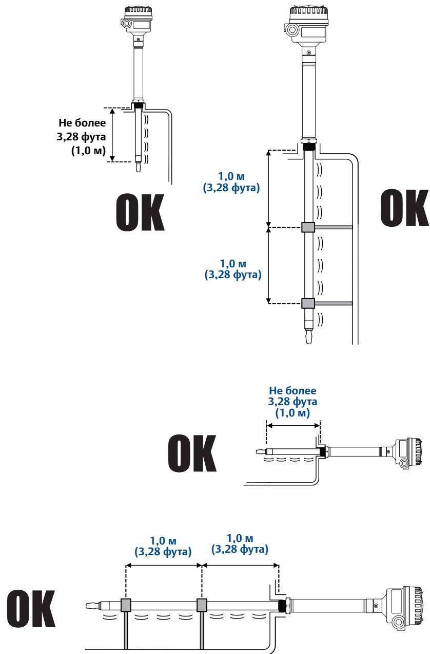
Рисунок 2-6. Монтаж удлиненной вилки на опоры (стандартный вариант)
