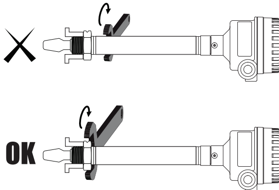
Рисунок 2-15. Затягивание сигнализатора 2130 с резьбовым соединением
