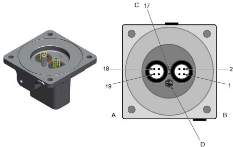
Рис. 12-2. Контакты гнезда адаптера датчика расхода
