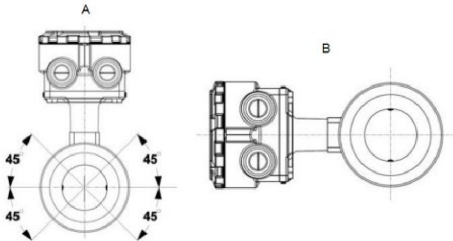
Рис. 3-4. Ориентация электродов
