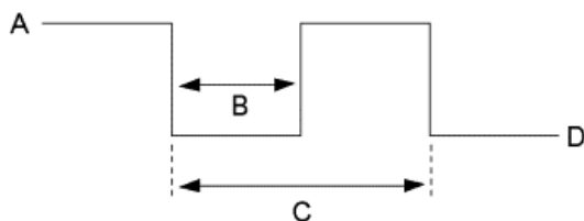
Рис. 8-1. Импульсный выход
