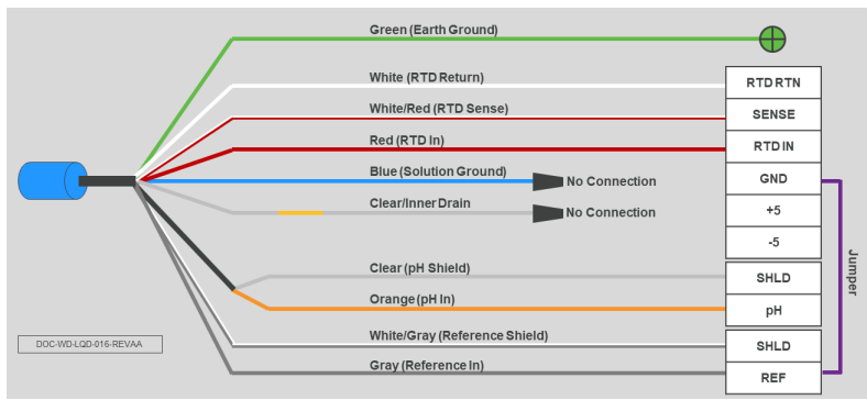
Рисунок 3-4. Подключение датчика pH/ОВП Rosemount 389VP, 396VP, 398VP или 398RVP без преусилителя к преобразователю Rosemount 56, 1056, 1057 или 1058
