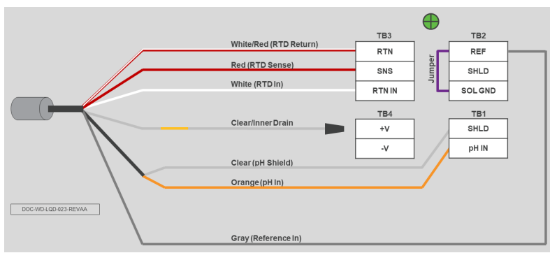
Рисунок 3-11. Подключение датчика рН/ОВП Rosemount 389, 396, 397, 398, или 398R без преусилителя к преобразователю Rosemount 1066
