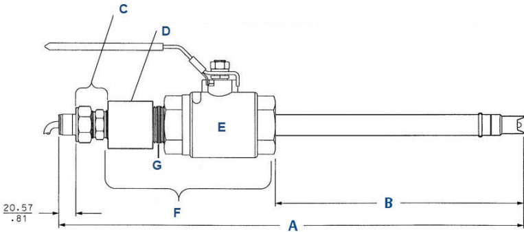
Рисунок 2-5. Шаровой клапан PN 23240-00 в сборе и переходник PN 23166-00 или PN 23166-01 с выдвигным датчиком Rosemount
