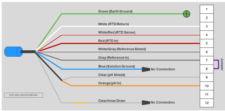
Рисунок 3-6. Подключение датчика рН/ОВП Rosemount 389VP, 396VP, 398VP или 398RVP без предусилителя к преобразователю Rosemount 5081
