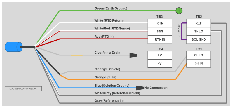
Рисунок 3-5. Подключение датчика pH/ОВП Rosemount 389VP, 396VP, 398VP или 398RVP без преусилителя к преобразователю Rosemount 1066
