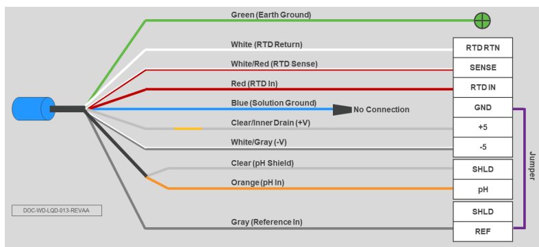
Рисунок 3-1. Подключение датчика Rosemount 389VP, 396VP или 398RVP с предусилителем к преобразователю Rosemount 56, 1056, 1057 или 1058
