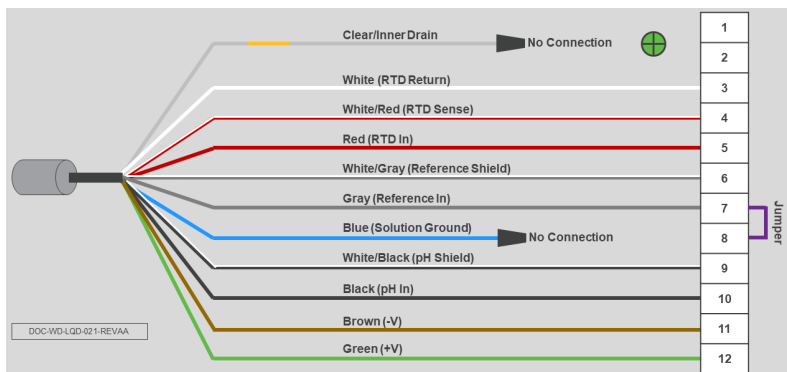
Рисунок 3-9. Подключение датчика pH/ОВП Rosemount 389 с предусилителем к измерительного преобразователю Rosemount 5081
