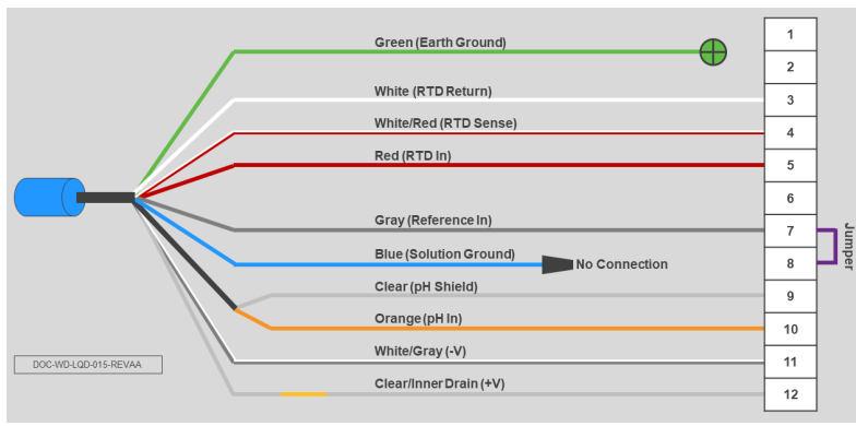
Рисунок 3-3. Подключение датчика рН/ОВП Rosemount 389VP, 396VP или 398RVP с предусилителем к преобразователю Rosemount 5081
