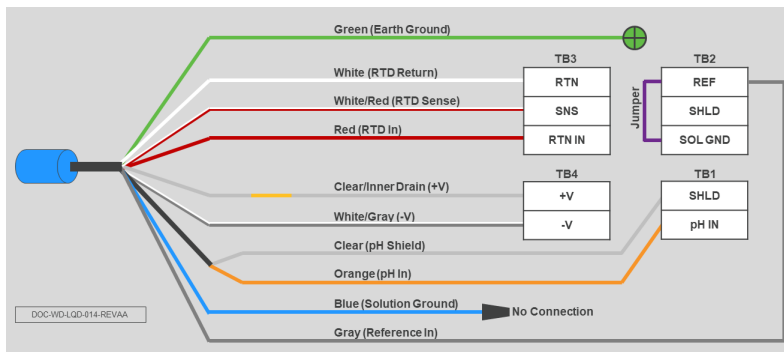
Рисунок 3-2. Подключение датчика рН/ОВП Rosemount 389VP, 396VP или 398RVP с предусилителем к преобразователю Rosemount 1066
