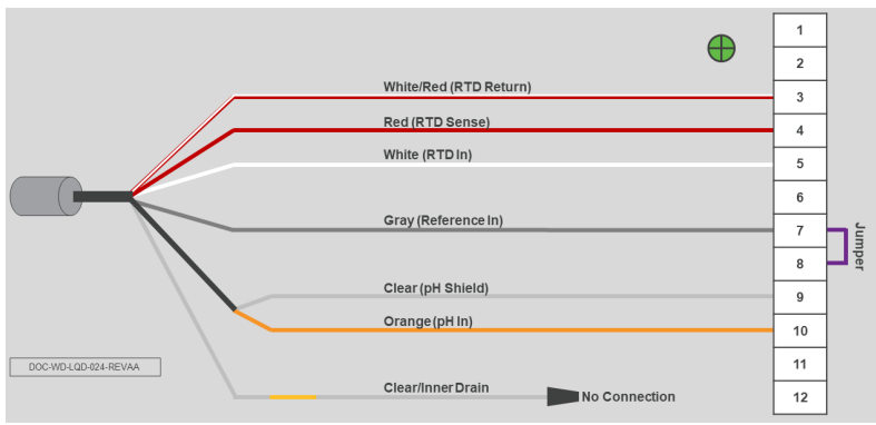
Рисунок 3-12. Подключение датчика рН/ОВП Rosemount 389, 396, 397, 398, или 398R без предусилителя к преобразователю Rosemount 5081
