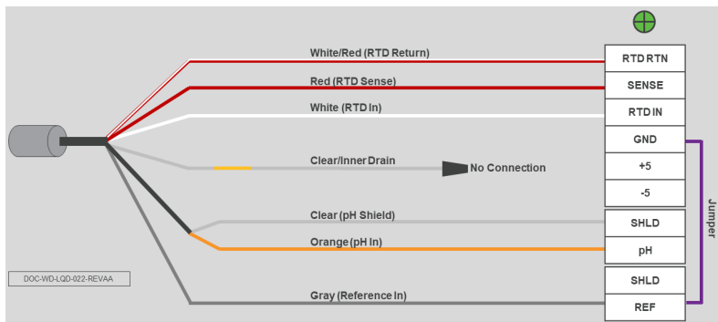
Рисунок 3-10. Подключение датчика рН/ОВП Rosemount 389, 396, 397, 398, или 398R без преусилителя к преобразователю Rosemount 56, 1056, 1057 или 1058
