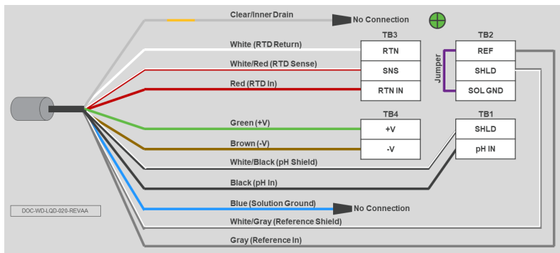
Рисунок 3-8. Подключение датчика pH/ОВП Rosemount 389 с предусилителем к измерительного преобразователю Rosemount 1066
