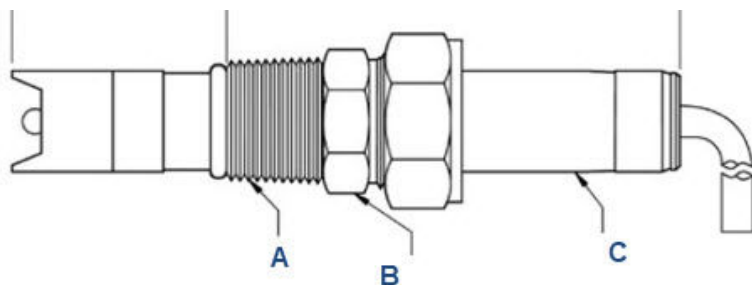
Рисунок 2-4. Переходник для установки (PN 23166-00 или PN 23166-01) с выдвижным датчиком Rosemount
