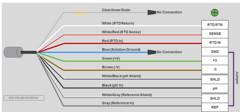
Рисунок 3-7. Подключение датчика рН/ОВП Rosemount 389 с предусилителем к преобразователю Rosemount 56, 1056, 1057 или 1058
