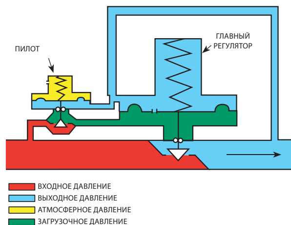
Рис.2. Регуляторы давления с пилотным приводом.
